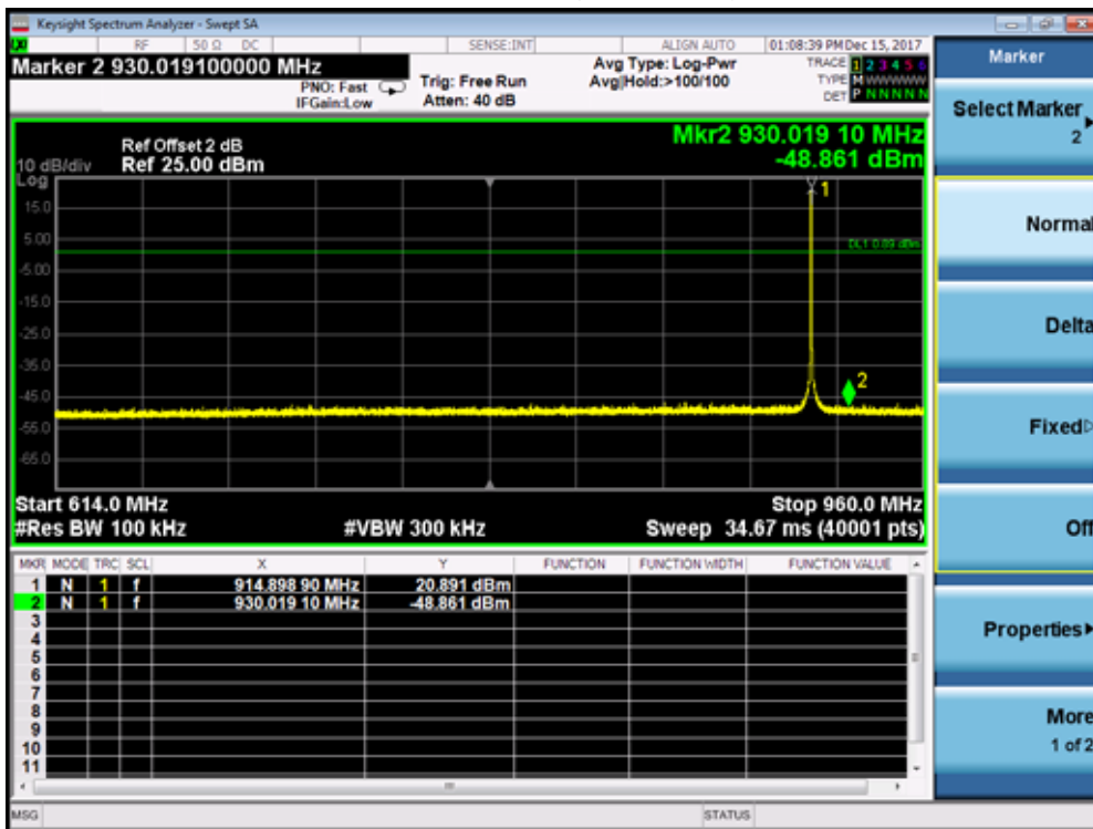
Mode 1 CH63(914.9MHz)
