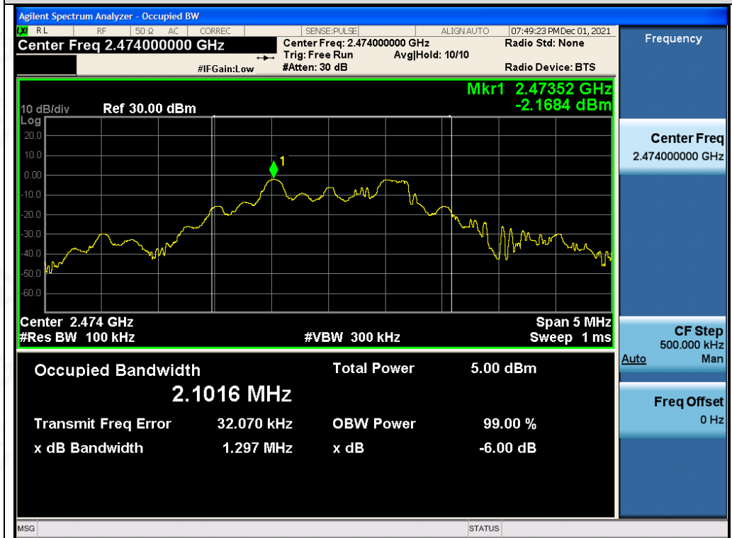
Test_Graph_FSK_ANT1_2474_DTSBW
