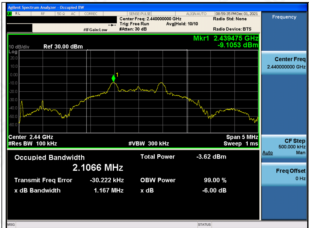
Test_Graph_FSK_ANT1_2440_DTSBW
