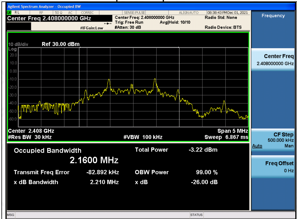
Test_Graph_FSK_ANT1_2408_OBW
