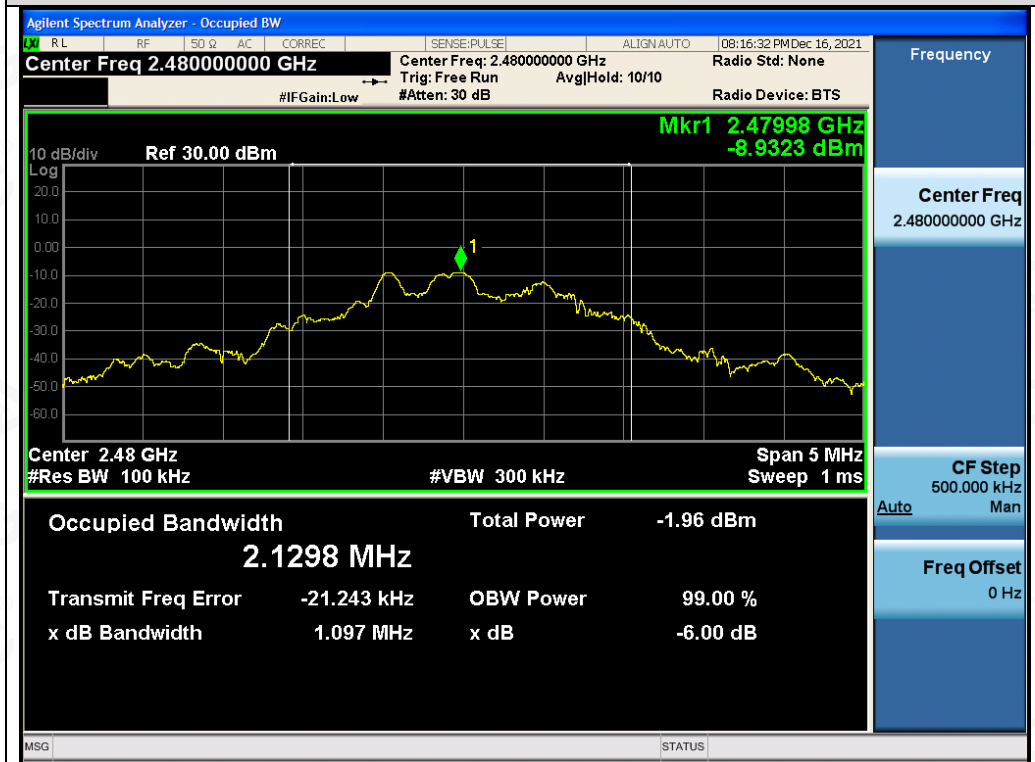
Test_Graph_FSK_ANT1_2480_DTBSBW
