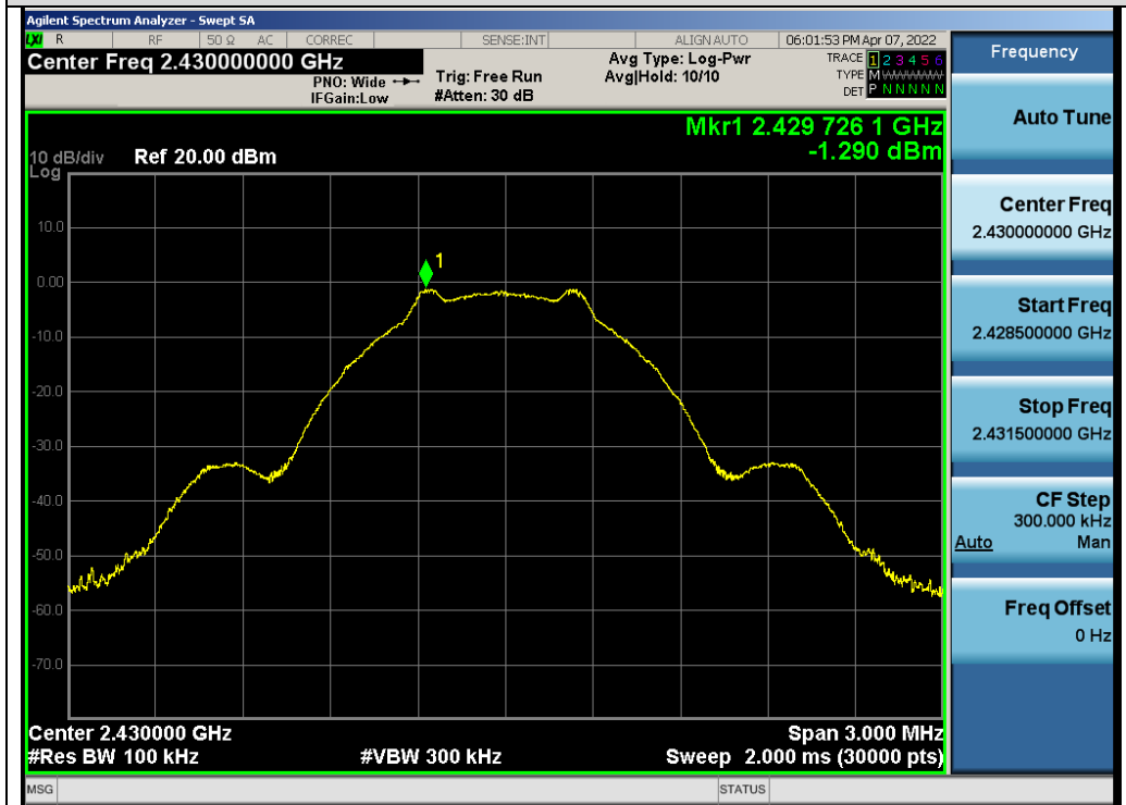
Test_Graph_GFSK_ANT1_2430_Reference Level
