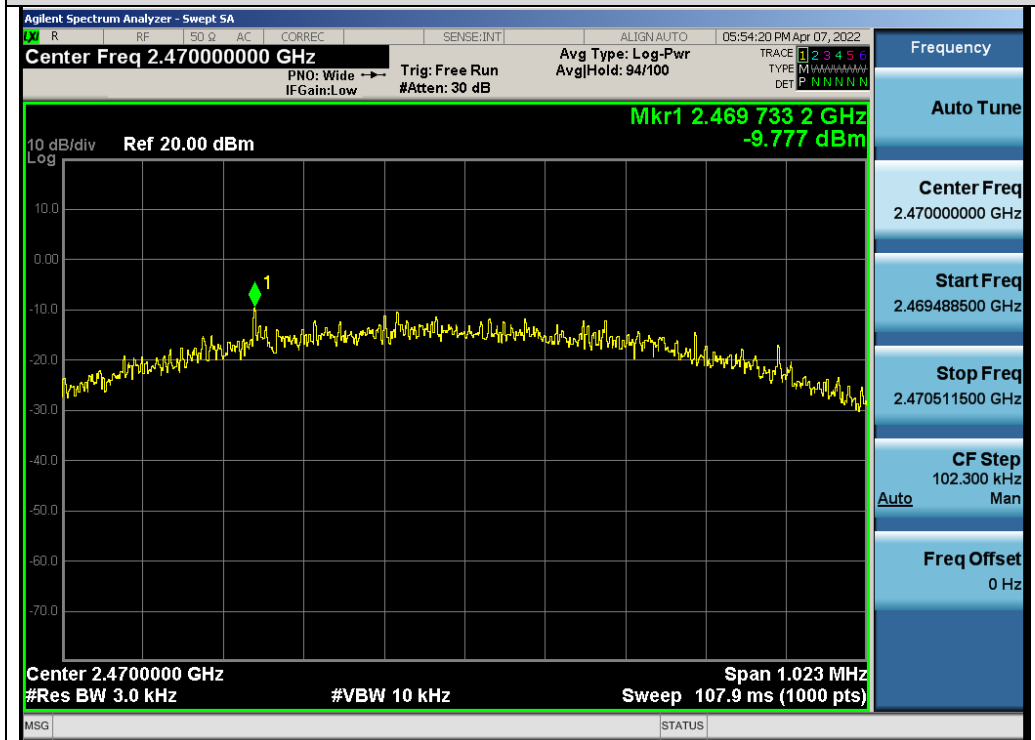
Test_Graph_GFSK_ANT1_2470_PSD
