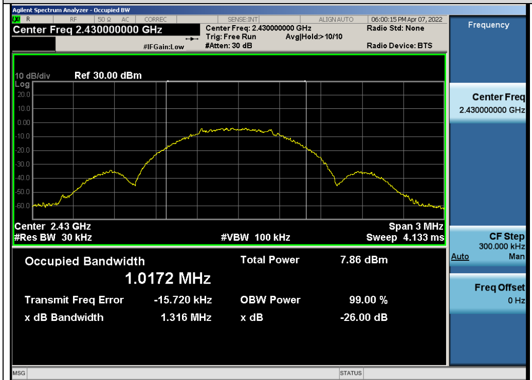
Test_Graph_GFSK_ANT1_2430_OBW
