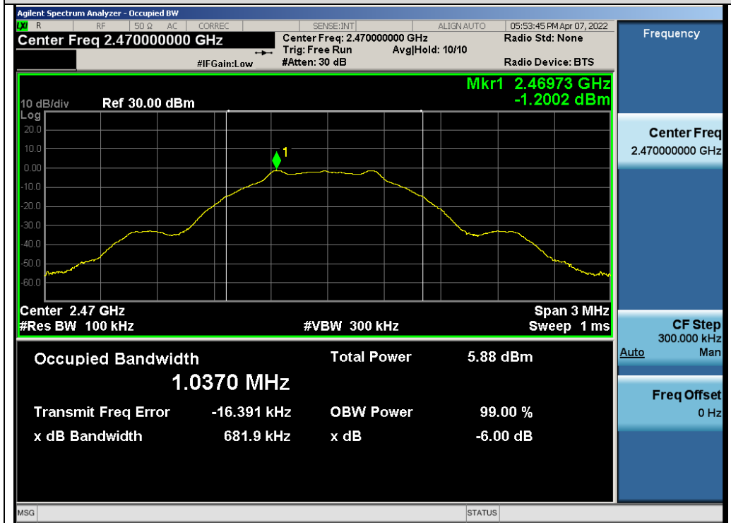
Test_Graph_GFSK_ANT1_2470_DTSBW
