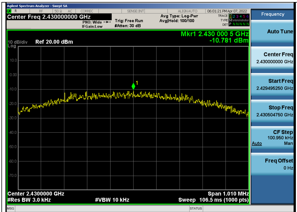
Test_Graph_GFSK_ANT1_2430_PSD
