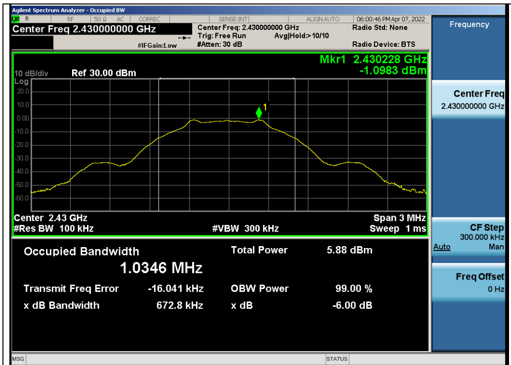
Test_Graph_GFSK_ANT1_2430_DTSBW
