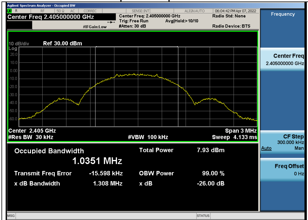
Test_Graph_GFSK_ANT1_2405_OBW
