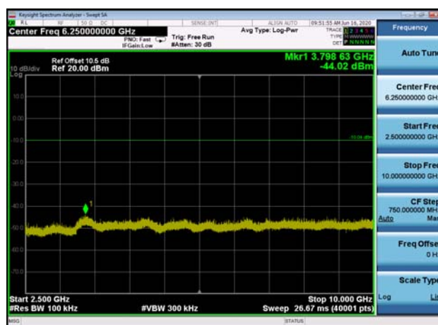
,Plot 4,2500MHz~10000MHz-802.11b ,2462MHz
