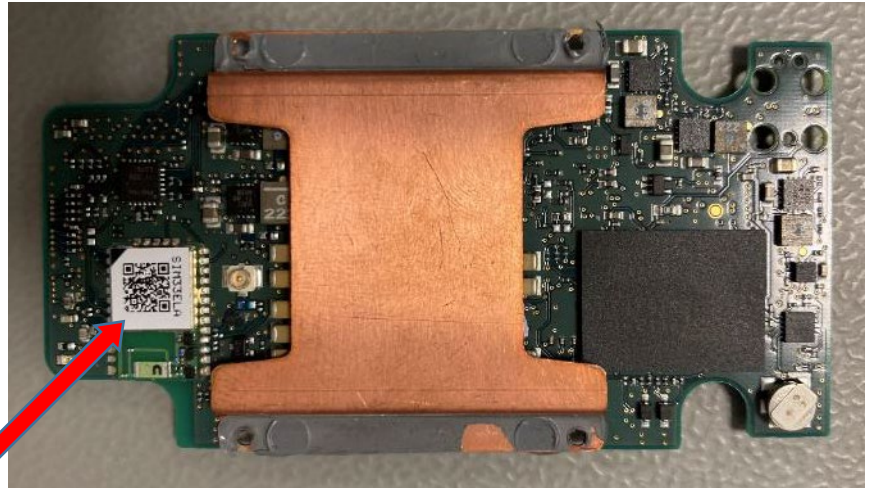
Mainboard PCB bottom
