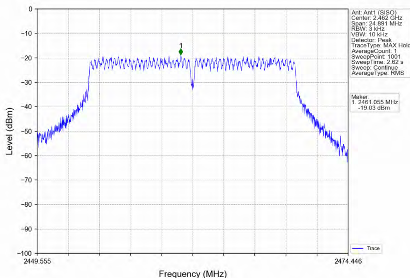
802.11g_HCH_2462MHz_Ant1 (SISO)_NTNV
