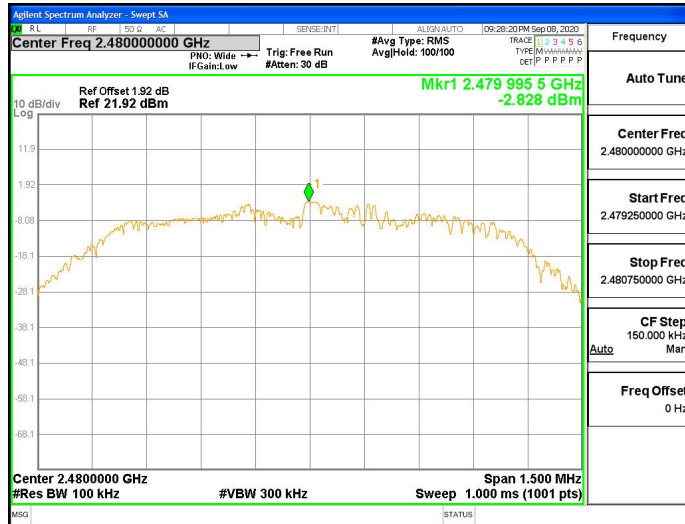
2DH1_Ant1_2480_30~100
