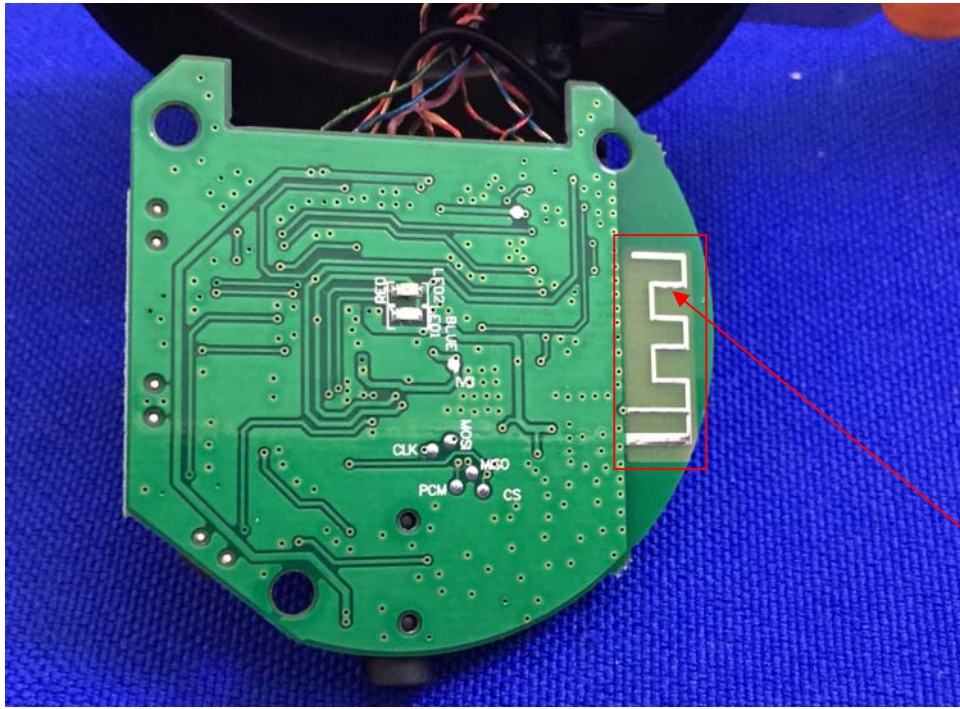
Antenna
