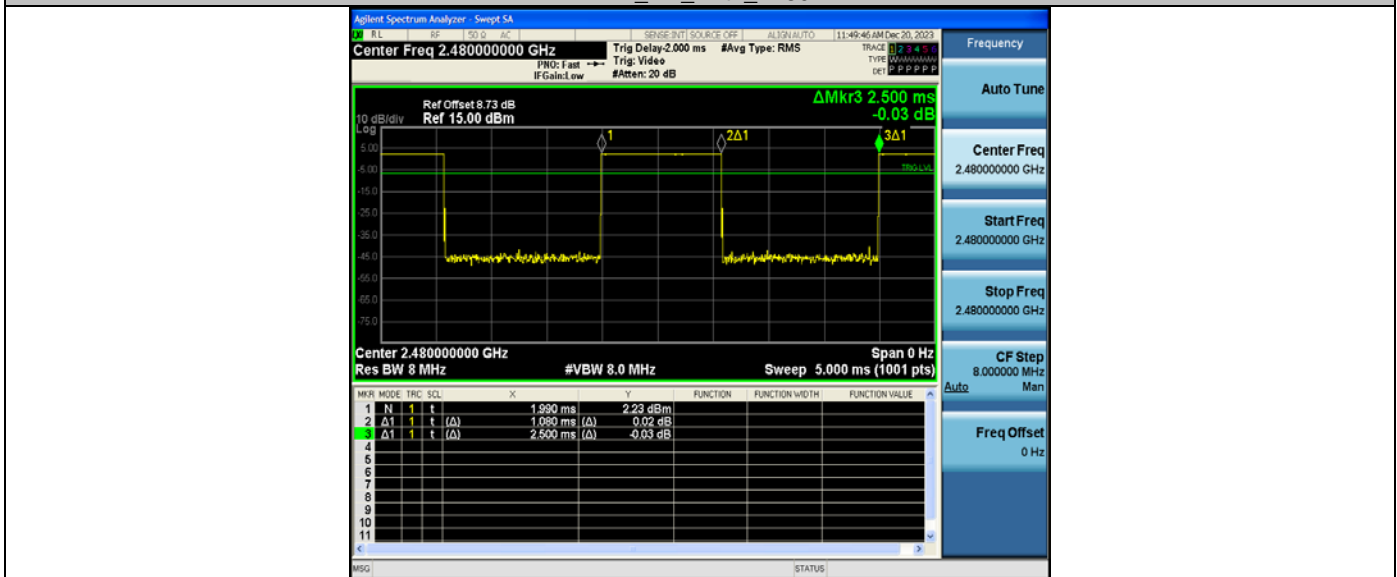
BLE_2M_Ant1_2480
