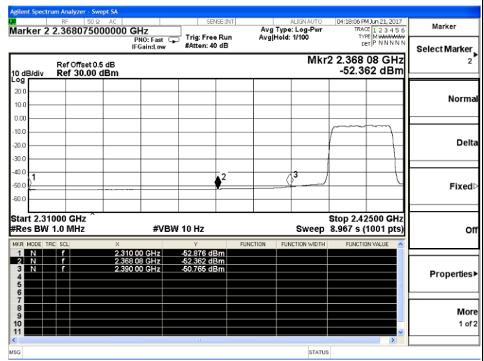
802.11n-HT20-Low channel(Average)
