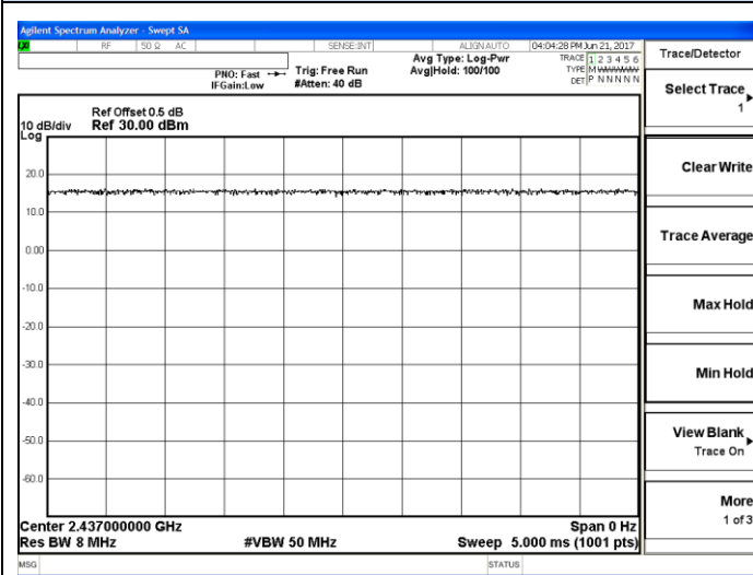
802.11n-HT20
