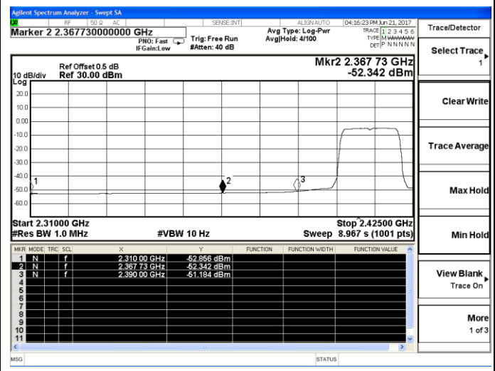
802.11g-Low channel(Average)
