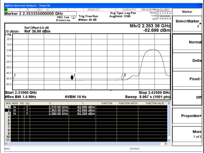
802.11b-Low channel(Average)
