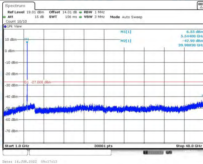
11AX40MIMO_Ant1_5550_1000~40000
