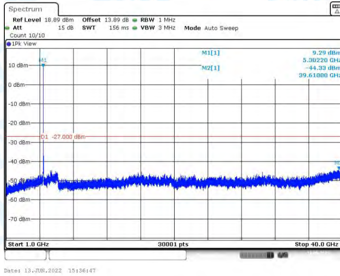
11AX20MIMO_Ant2_5300_1000~40000
