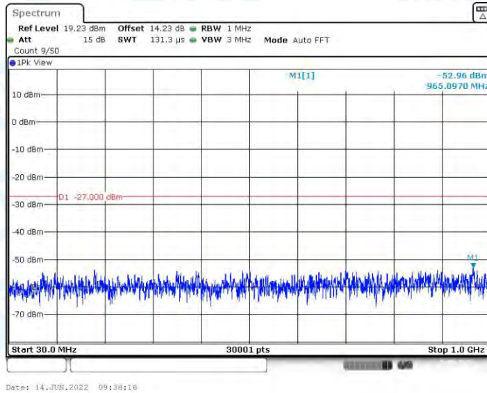
11AX40MIMO_Ant2_5670_30~1000
