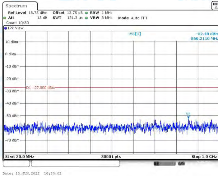
11AX40MIMO_Ant2_5310_30~1000
