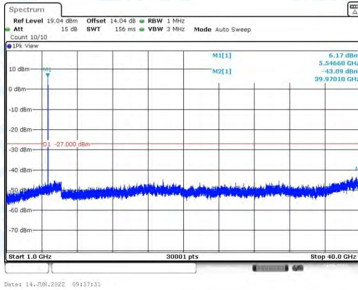
11AX40MIMO_Ant2_5550_1000~40000
