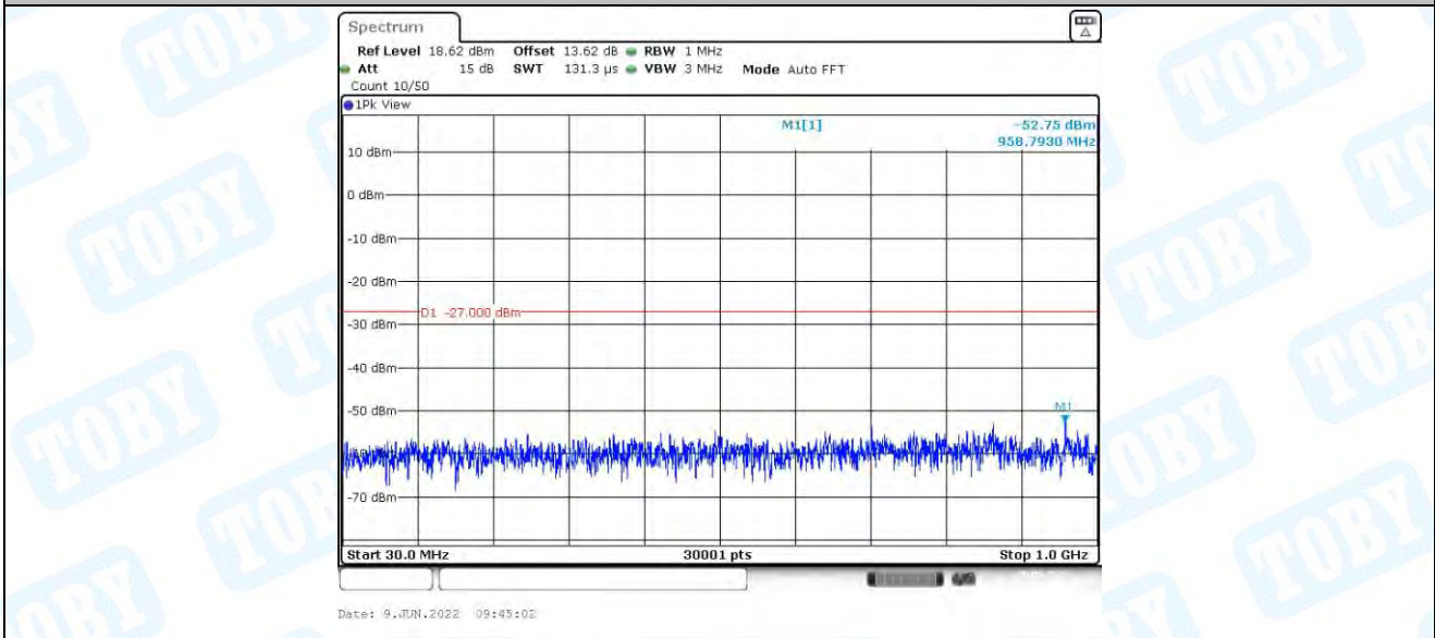
11AX20MIMO_Ant2_5220_30~1000
