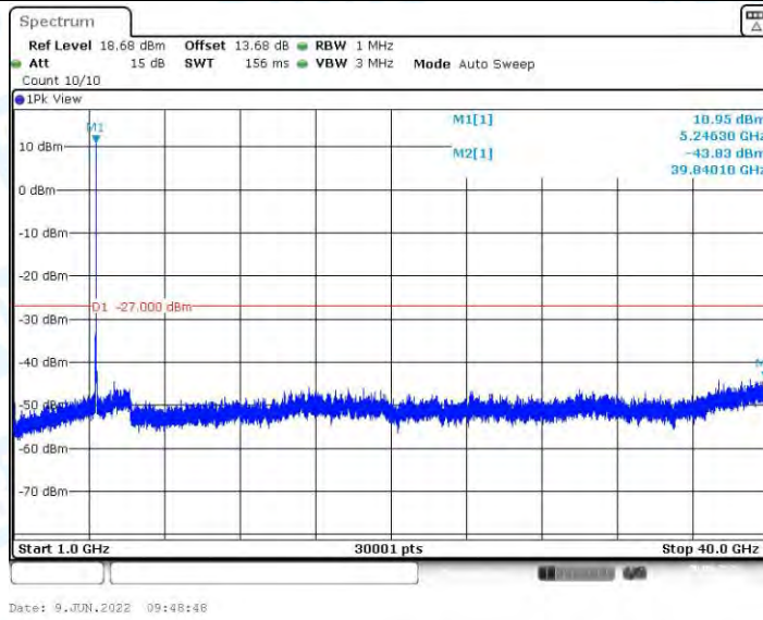
11AX20MIMO_Ant1_5240_1000~40000
