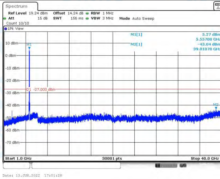
11AX80MIMO_Ant1_5530_1000~40000
