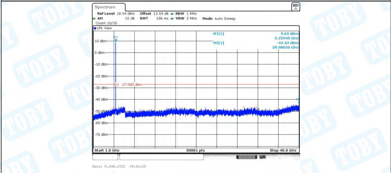
11AX20MIMO_Ant1_5220_1000~40000
