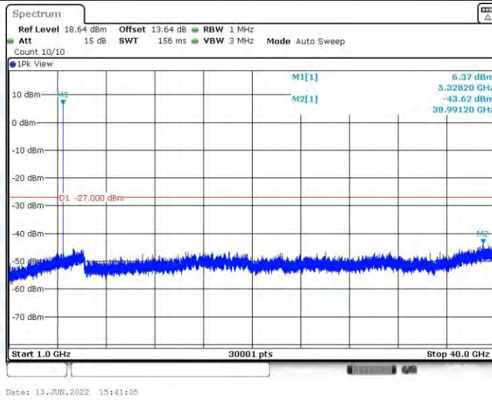
11AX20MIMO_Ant1_5320_1000~40000
