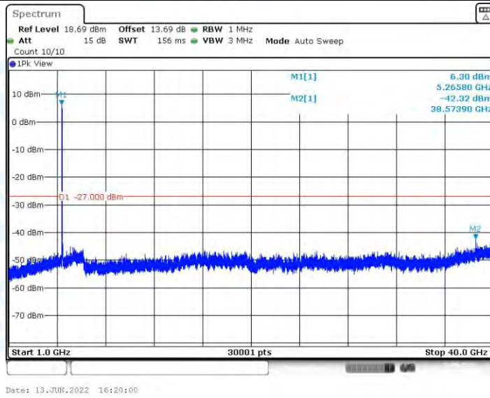
11AX40MIMO_Ant1_5270_1000~40000
