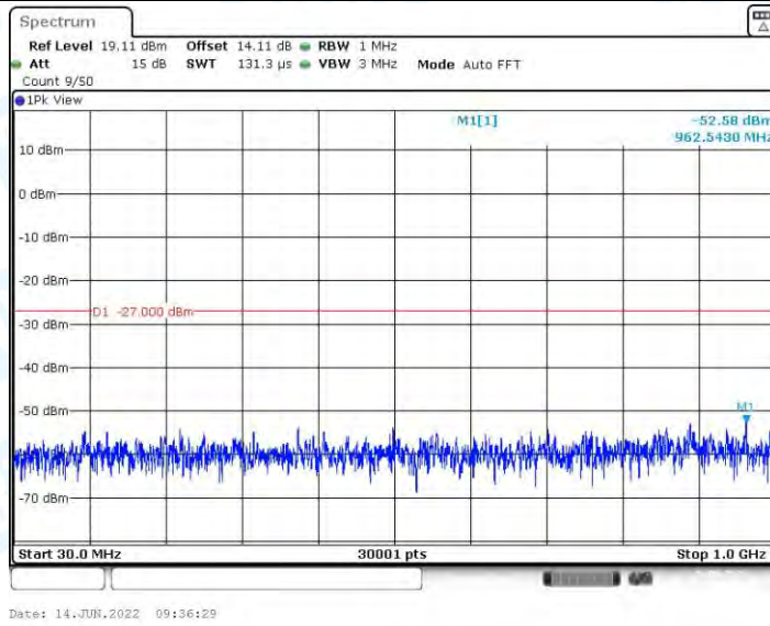
11AX40MIMO_Ant2_5510_30~1000
