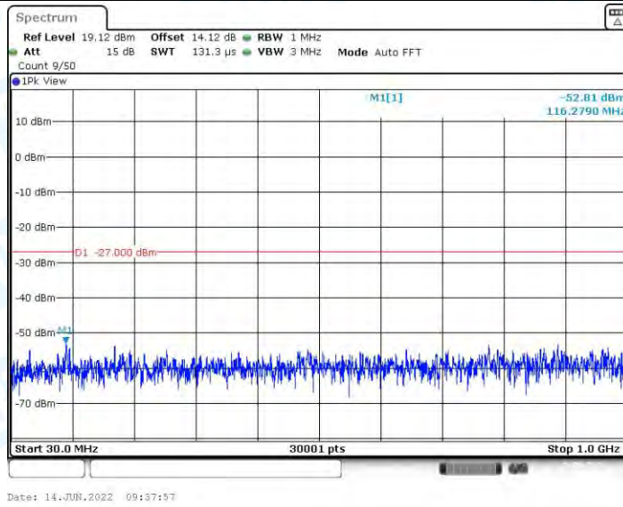
11AX40MIMO_Ant1_5670_30~1000
