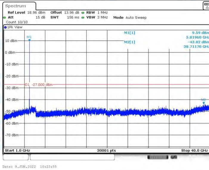
11AX20MIMO_Ant1_5825_1000~40000
