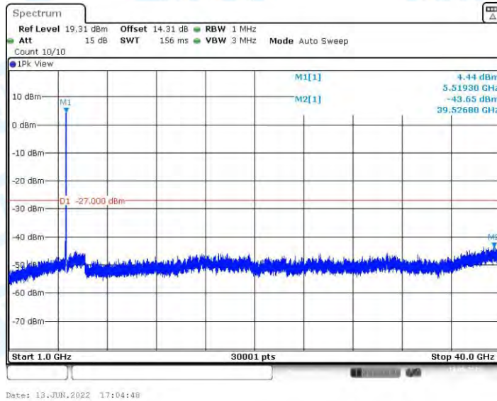
11AX80MIMO_Ant2_5530_1000~40000
