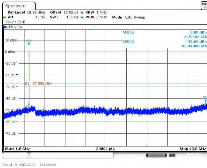
11AX40MIMO_Ant1_5795_1000~40000
