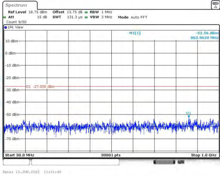
11N20MIMO_Ant1_5260_30~1000
