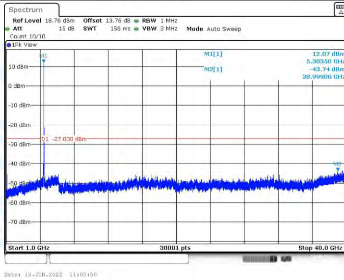
11N20MIMO_Ant1_5300_1000~40000
