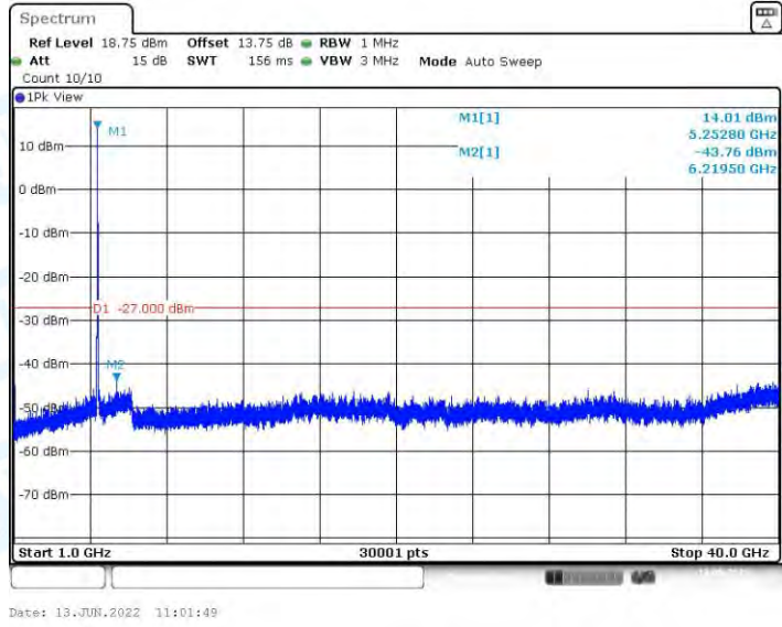
11N20MIMO_Ant1_5260_1000~40000
