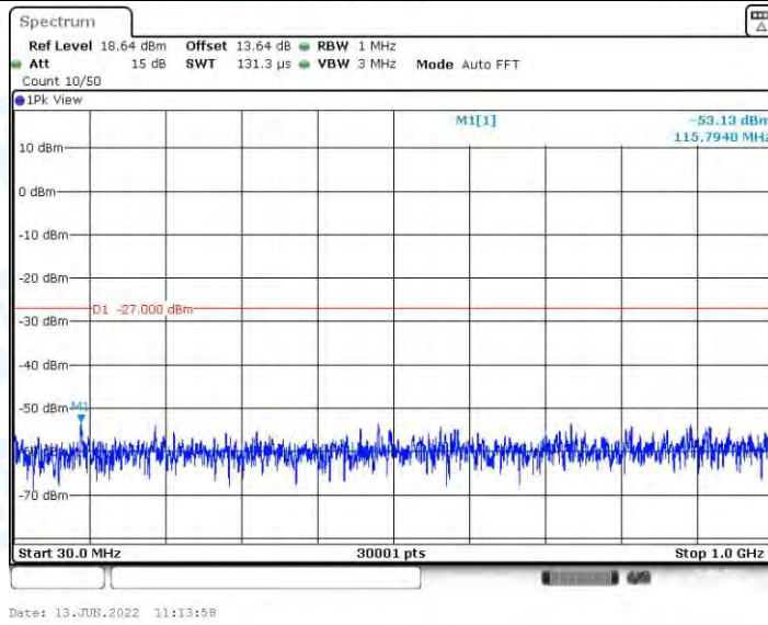
11N20MIMO_Ant1_5320_30~1000
