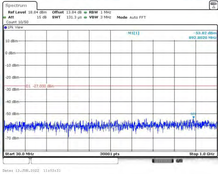
11N20MIMO_Ant2_5260_30~1000
