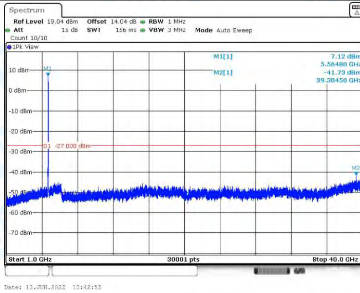
11N40MIMO_Ant2_5550_1000~40000
