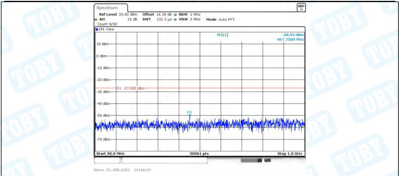
11N20MIMO_Ant2_5300_30~1000
