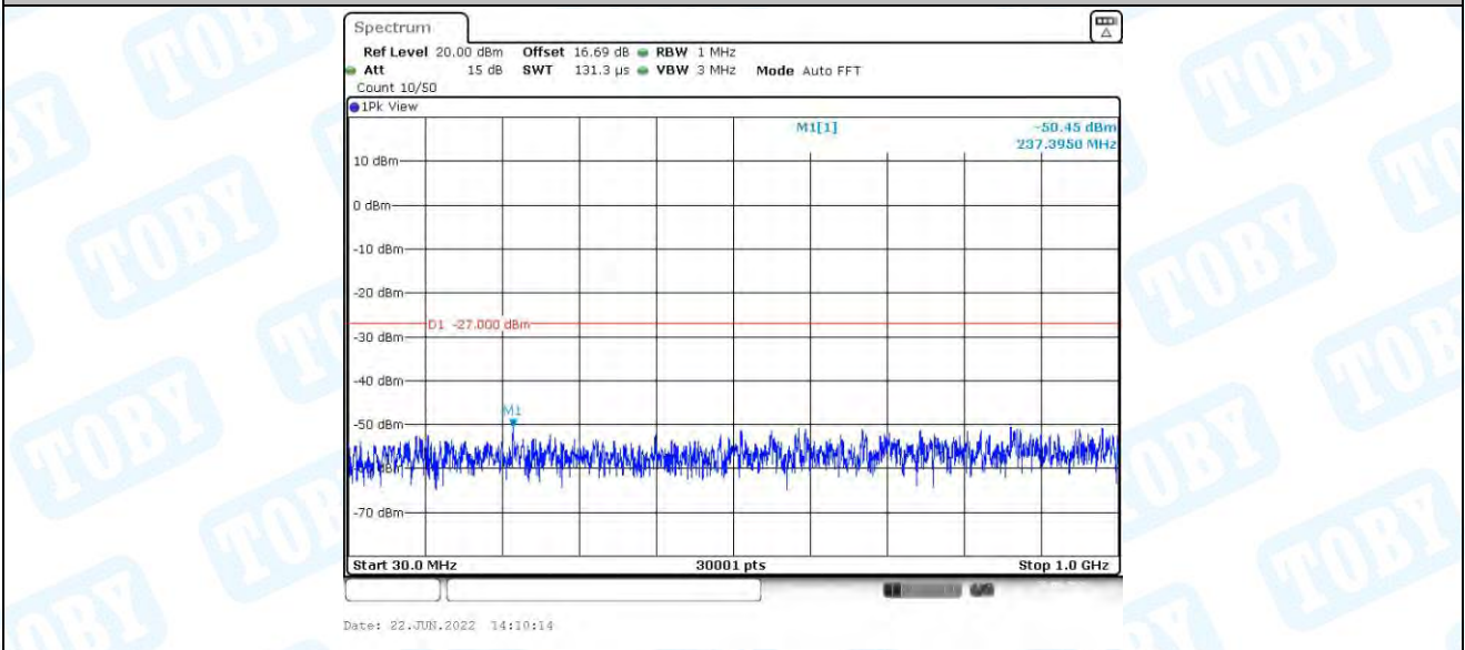
11AC20MIMO_Ant1_5700_30~1000
