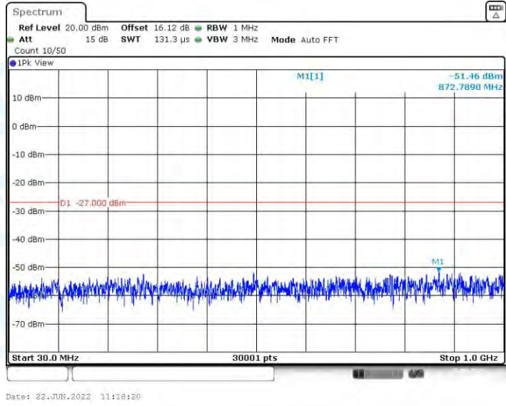
11AC20MIMO_Ant2_5220_30~1000
