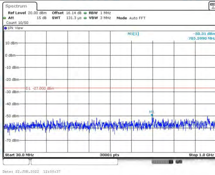
11AC20MIMO_Ant1_5320_30~1000
