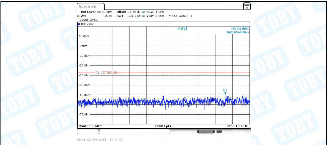
11N40MIMO_Ant1_5670_30~1000
