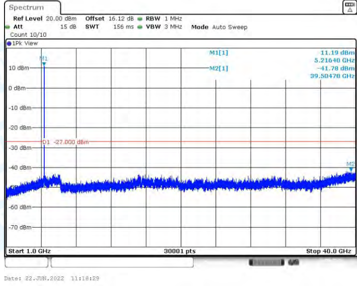
11AC20MIMO_Ant2_5220_1000~40000
