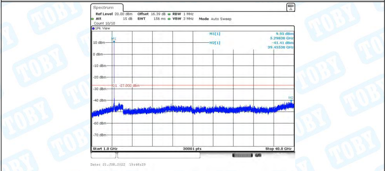
11N20MIMO_Ant2_5300_1000~40000
