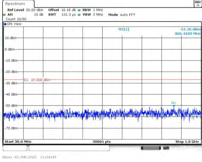
11AC20MIMO_Ant1_5240_30~1000
