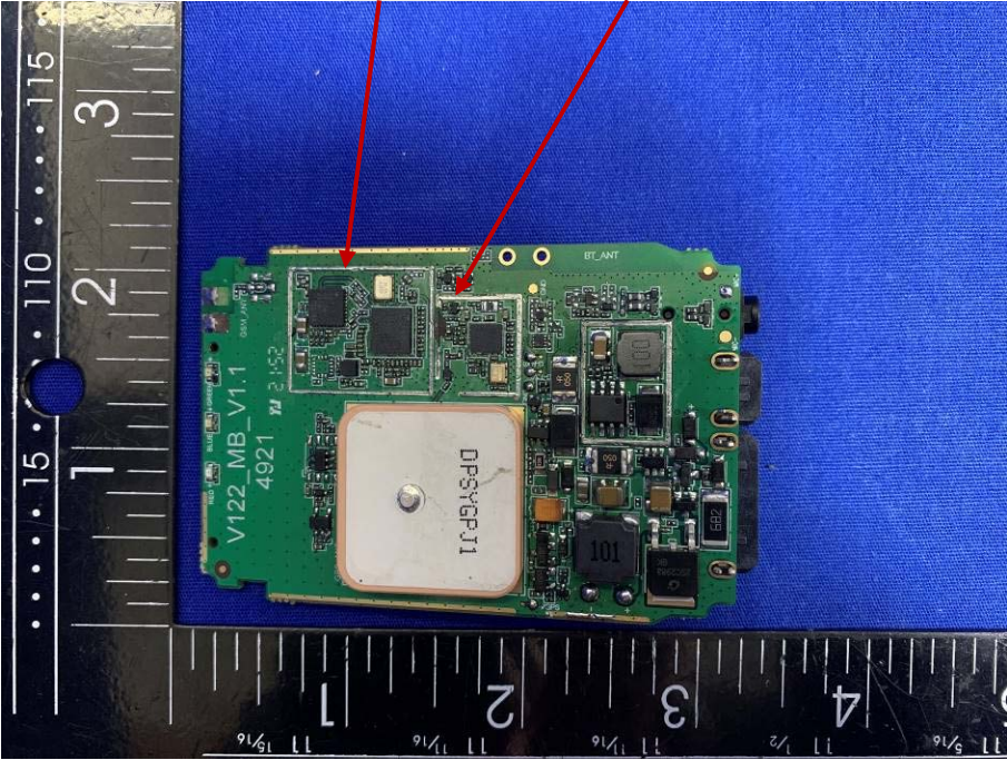
GSM Module GPS Module
