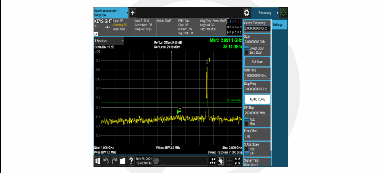
Band7-20MHz-QPSK-20850-100RB#0-Range1:1000~3000MHz
