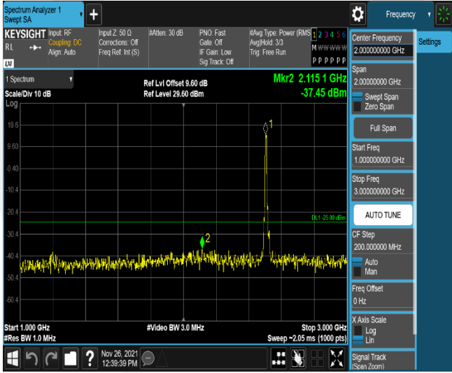
Band7-20MHz-QPSK-21100-100RB#0-Range 1:1000~3000MHz
