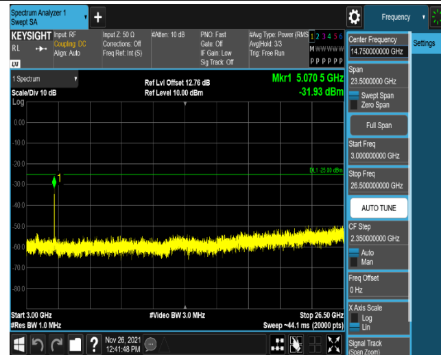
Band7-20MHz-QPSK-21350-100RB#0-Range1:3000~26500MHz
