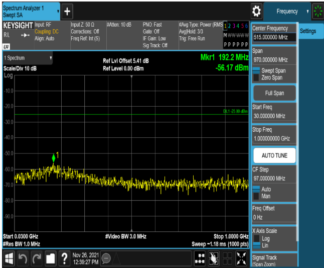
Band7-20MHz-QPSK-21100-100RB#0-Range 1:30~1000MHz
