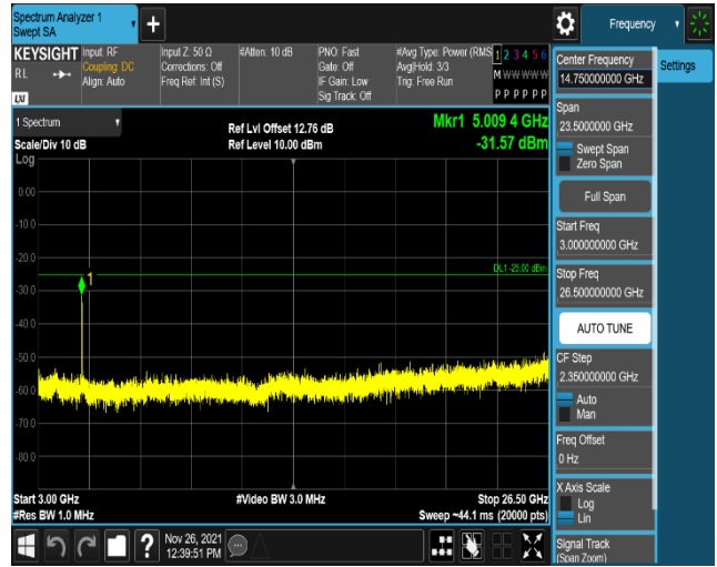
Band7-20MHz-QPSK-21100-100RB#0-Range 1:3000~26500MHz
