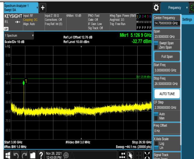
Band7-20MHz-16QAM -21100-100RB#0-Range1:3000~26500MHz
