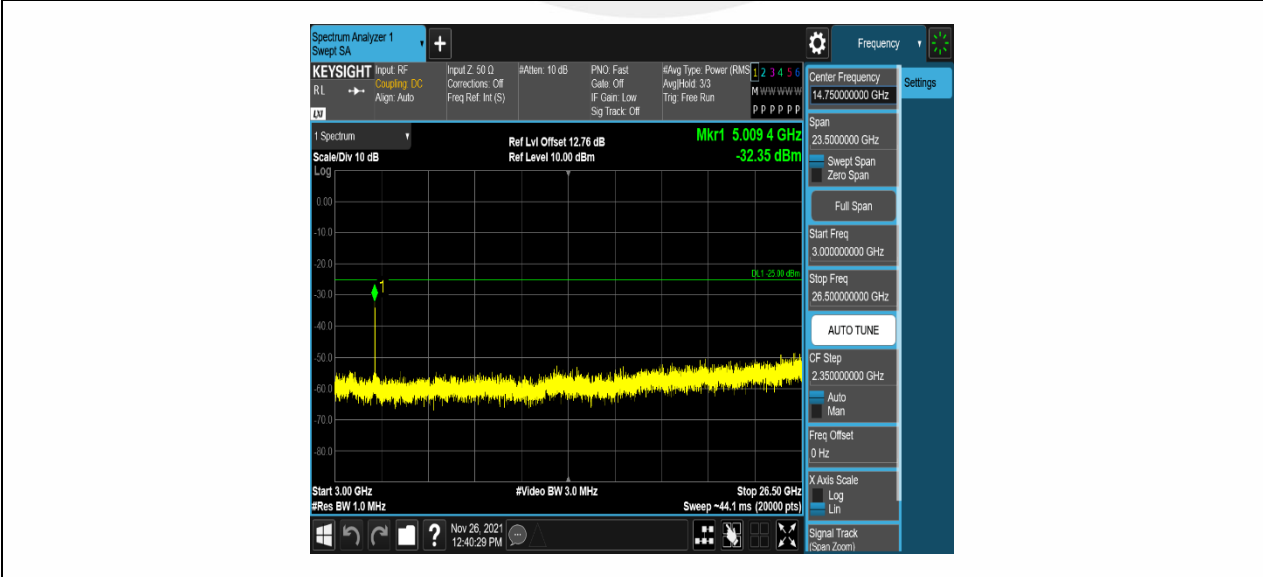
Band7-20MHz-QPSK-20850-100RB#0-Range1:3000~26500MHz
