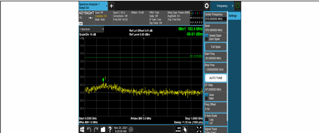
Band7-10MHz-QPSK-20800-50RB#0-Range1:30~1000MHz
