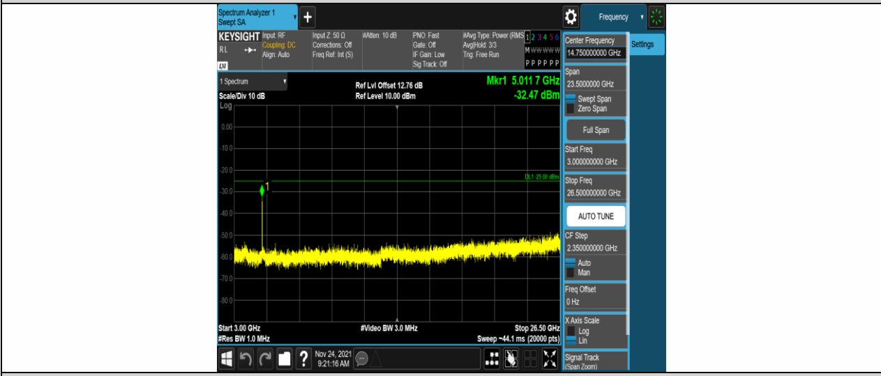
Band7-10MHz-QPSK-20800-50RB#0-Range3:3000~26500MHz
