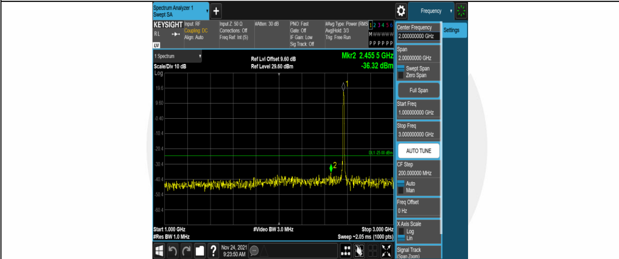
Band7-10MHz-QPSK-21400-50RB#0-Range2:1000~3000MHz
