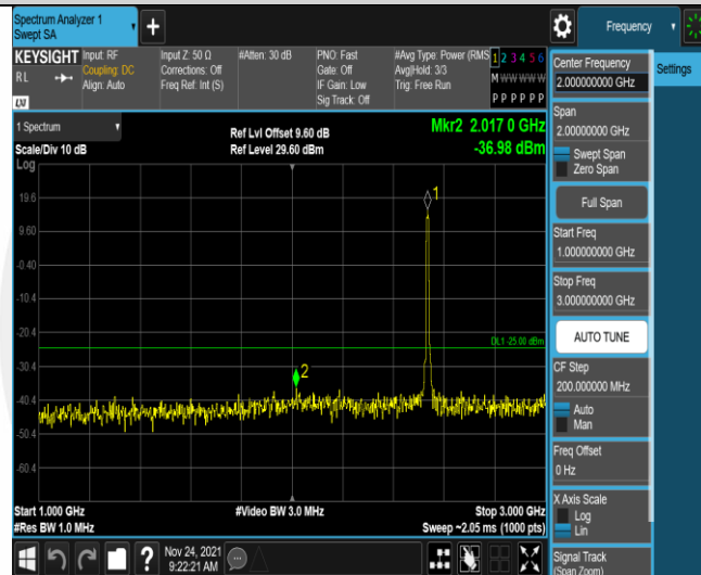
Band7-10MHz-QPSK-21100-50RB#0-Range2:1000~3000MHz
