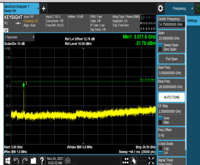
Band7-10MHz-QPSK-21100-50RB#0-Range3:3000~26500MHz
