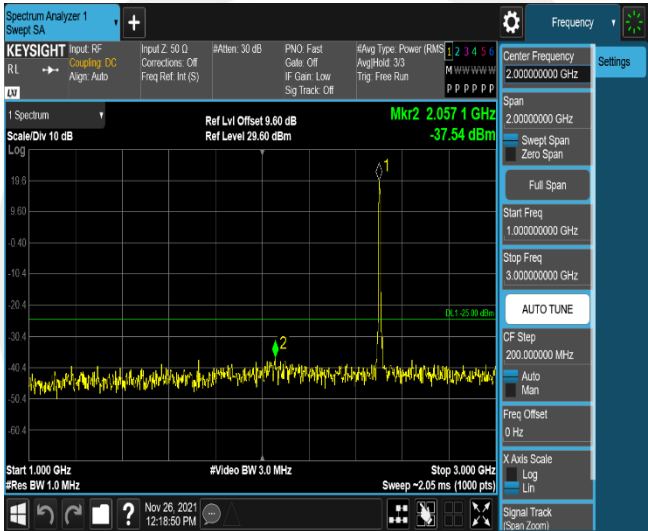
Band7-10MHz-16QAM-21100-50RB#0-Range2:1000~3000MHz
