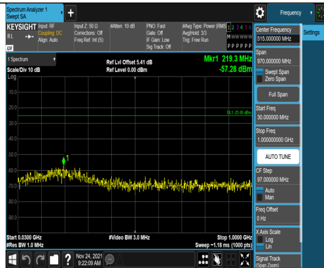
Band7-10MHz-QPSK-21100-50RB#0-Range1:30~1000MHz
