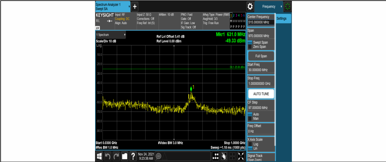
Band7-10MHz-QPSK-21400-50RB#0-Range1:30~1000MHz
