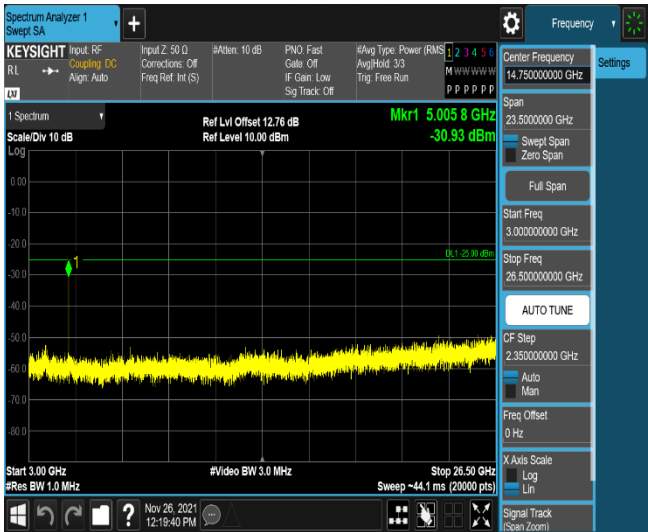
Band7-10MHz-16QAM-20800-50RB#0-Range3:3000~26500MHz
