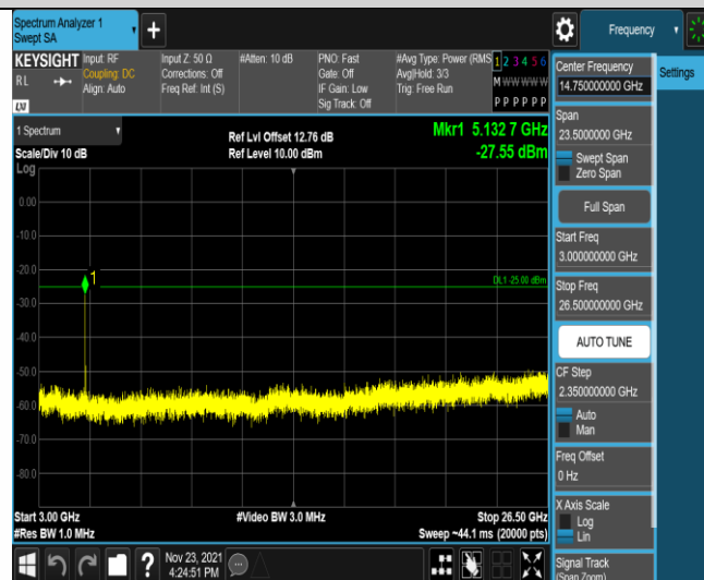
Band7-5MHz-QPSK-21425-25RB#0-Range3:3000~26500MHz
