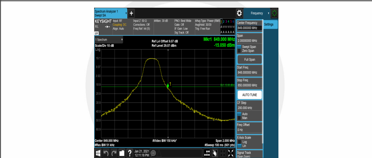
Band5-3MHz-QPSK-20635-1RB#14
