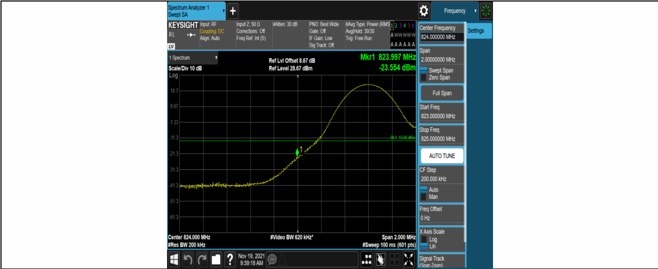
Band5-10MHz-QPSK-20450-1RB#0
