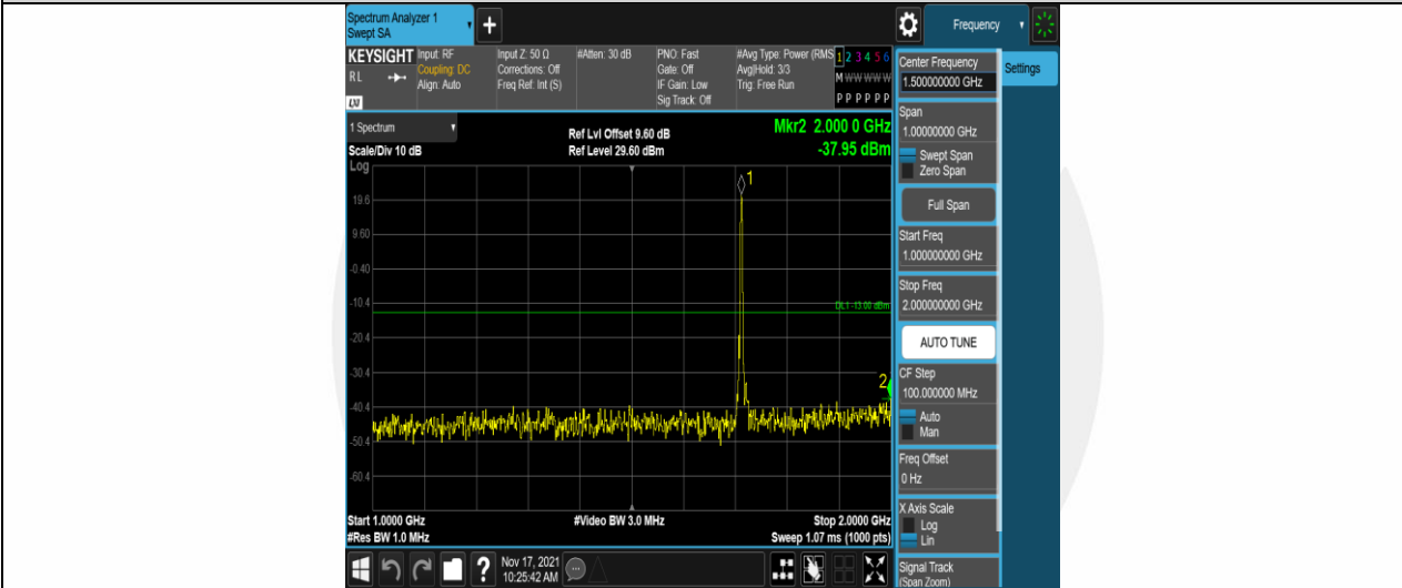
Band4-3MHz-QPSK-19965-1RB#0-Range2:1000~2000MHz
