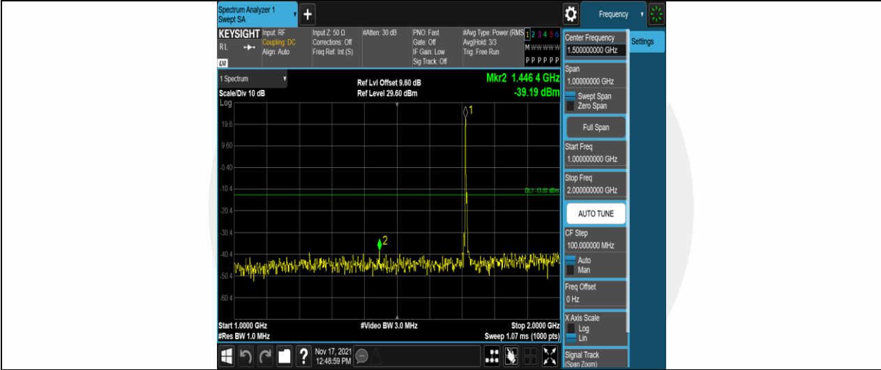
Band4-5MHz-QPSK-19975-1RB#0-Range2:1000~2000MHz
