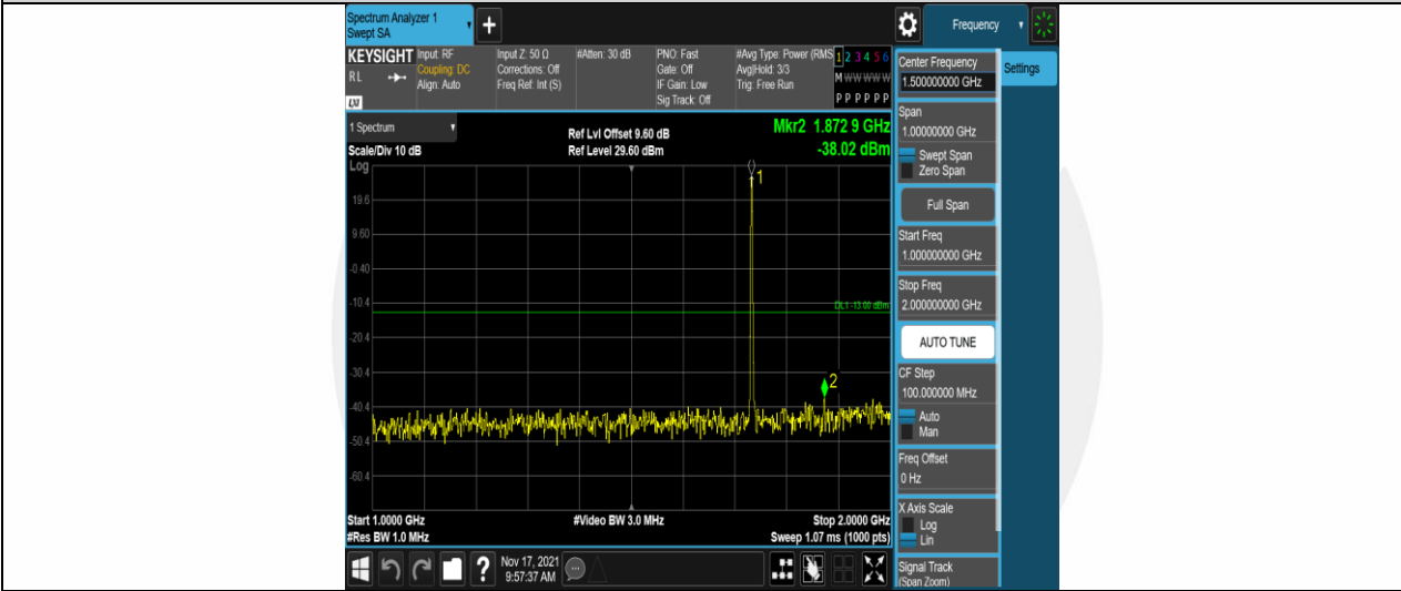
Band4-1.4MHz-QPSK-20175-1RB#0-Range2:1000~2000MHz
