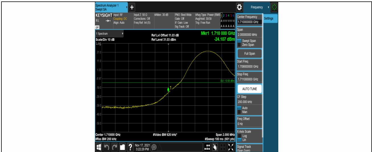
Band4-10MHz-QPSK-20000-1RB#0
