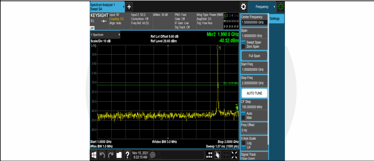
Band2-5MHz-QPSK-18625-1RB#0-Range2:1000~2000MHz
