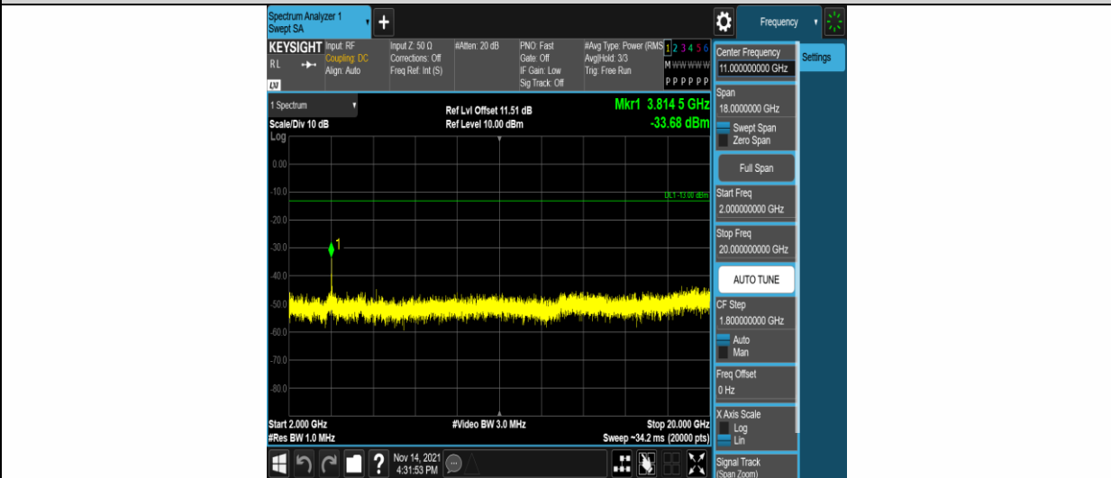
Band2-3MHz-QPSK-19185-1RB#0-Range3:2000~20000MHz
