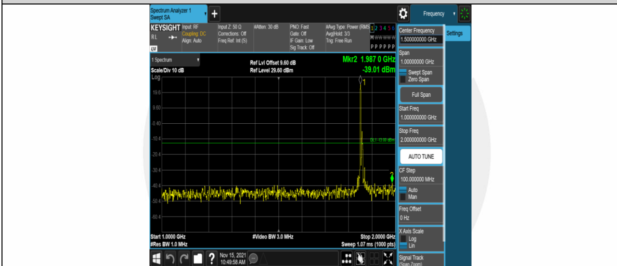
Band2-10MHz-QPSK-18650-1RB#0-Range2:1000~2000MHz
