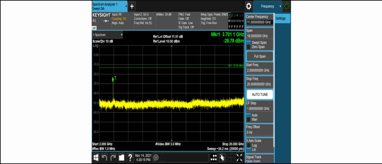
Band2-3MHz-QPSK-18615-1RB#0-Range3:2000~20000MHz
