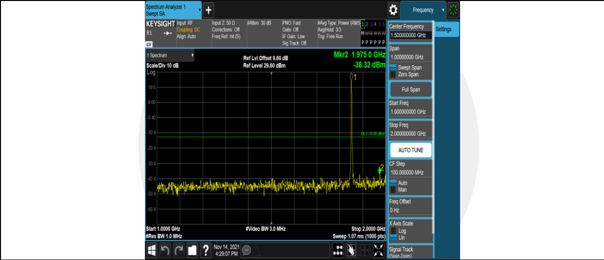
Band2-3MHz-QPSK-18615-1RB#0-Range2:1000~2000MHz
