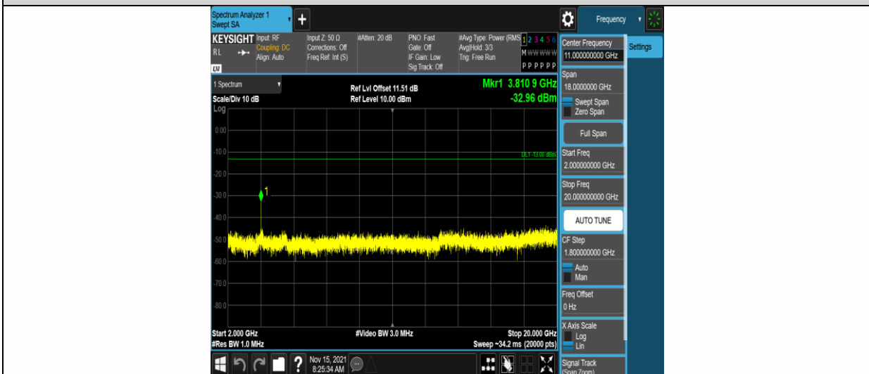
Band2-5MHz-QPSK-19175-1RB#0-Range3:2000~20000MHz
