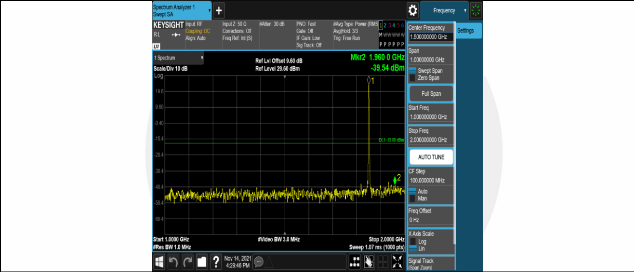
Band2-3MHz-16QAM-18615-1RB#0-Range2:1000~2000MHz
