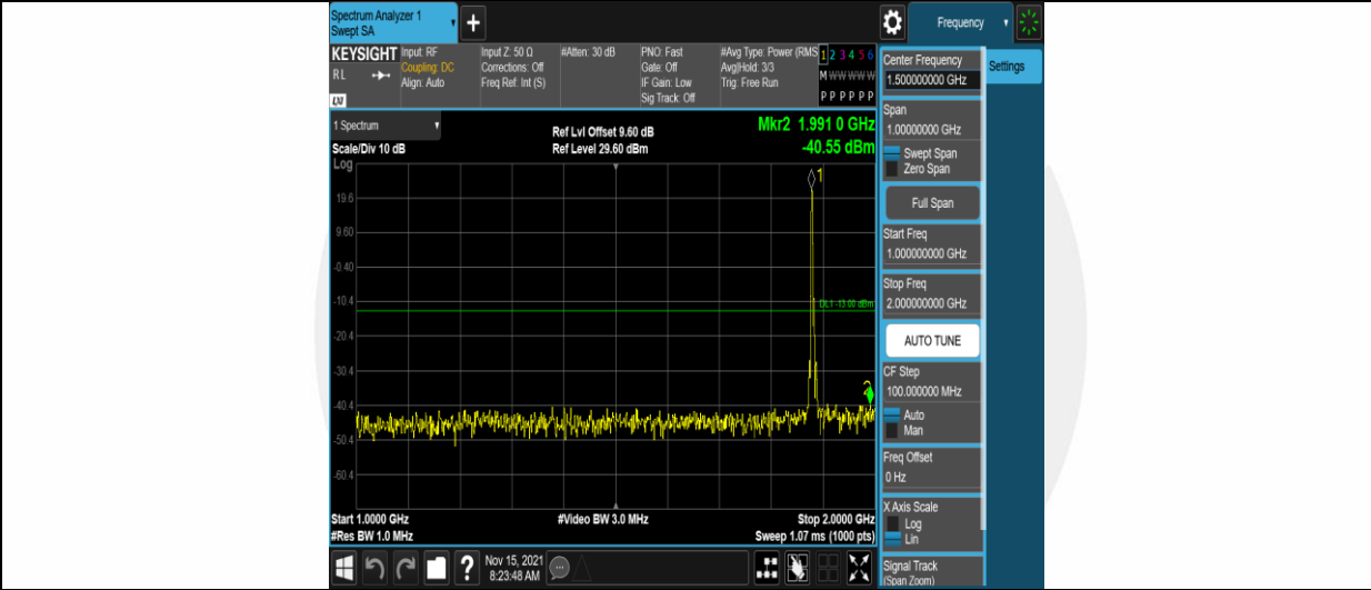
Band2-5MHz-QPSK-18900-1RB#0-Range2:1000~2000MHz
