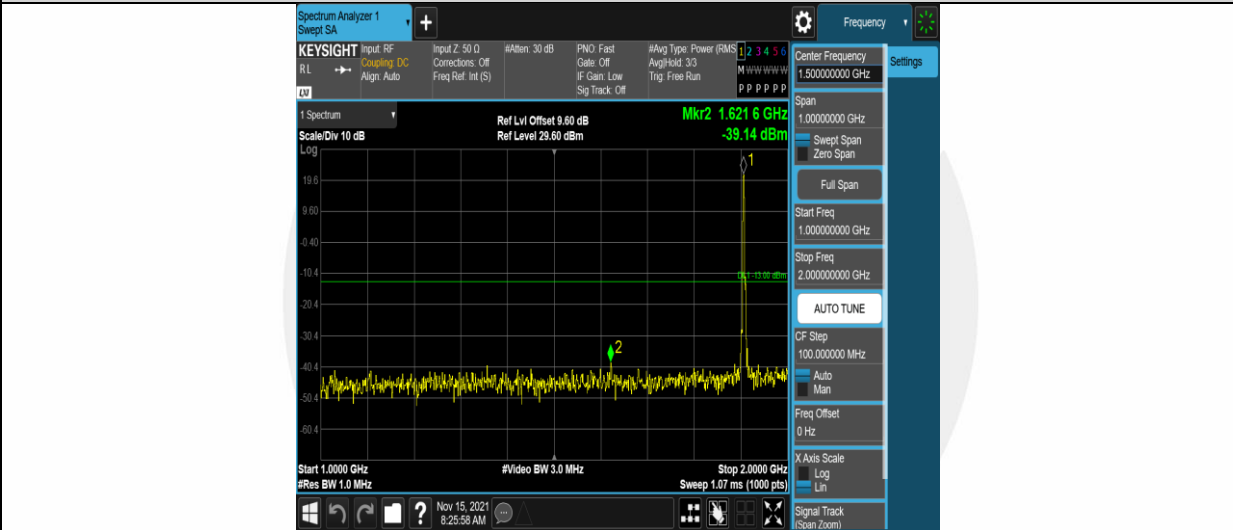
Band2-5MHz-16QAM-19175-1RB#0-Range2:1000~2000MHz
