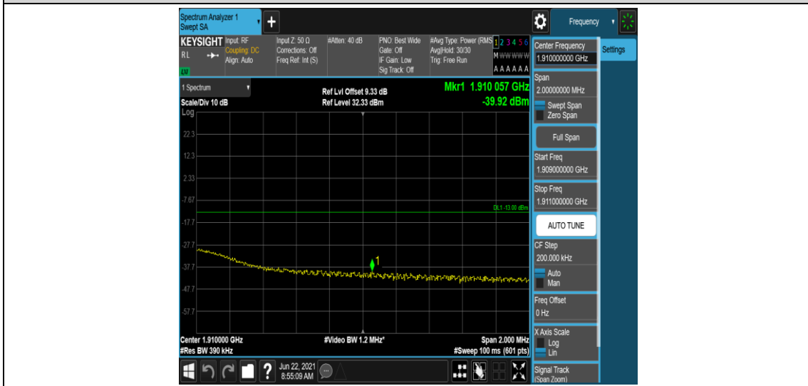
Band2-20MHz-16QAM-19100-1RB#99
