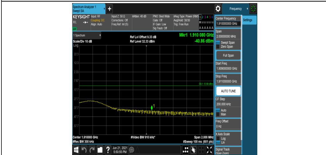
Band2-15MHz-16QAM-19125-1RB#74
