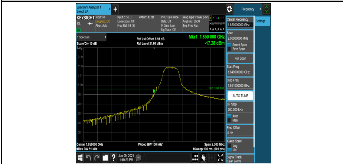
Band2-3MHz-QPSK-18615-1RB#14
