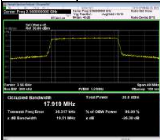
16QAM-21100
