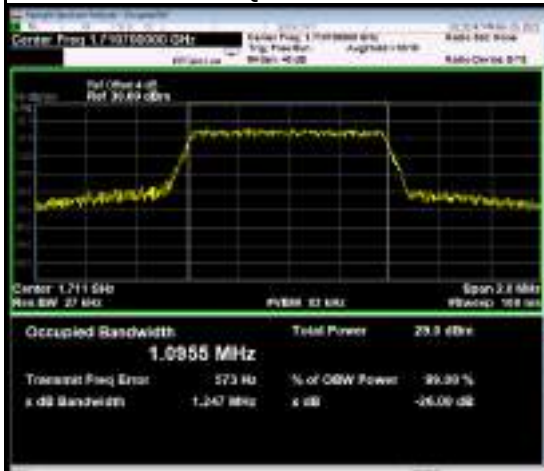
QPSK-132665
