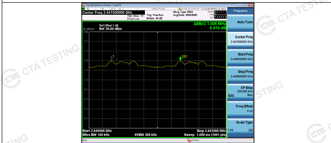
\pi/4 DQPSK
