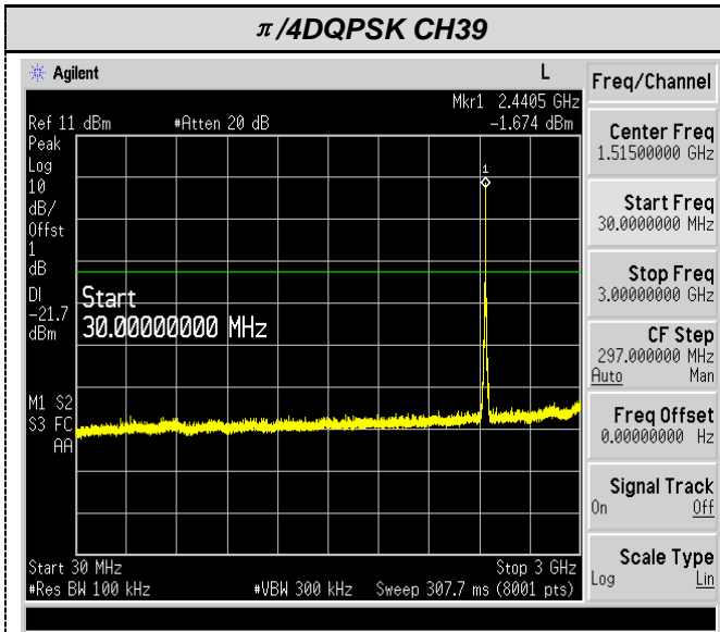
30MHz-3GHz
