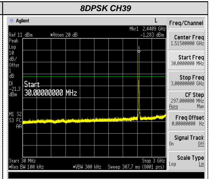
30MHz-3GHz
