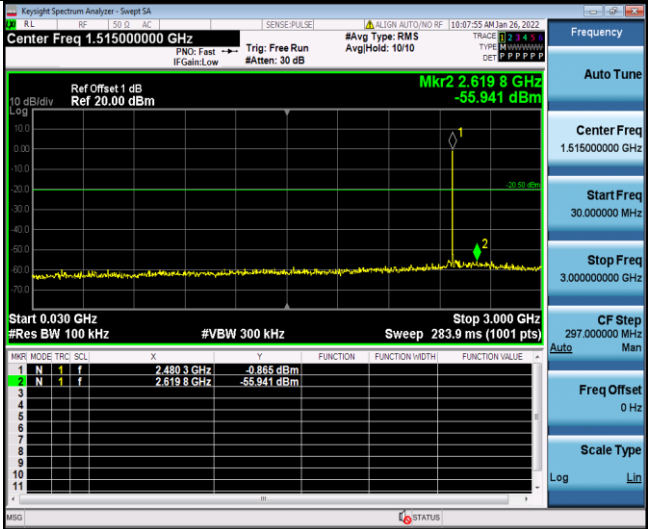
BLE 2480 30-3000
