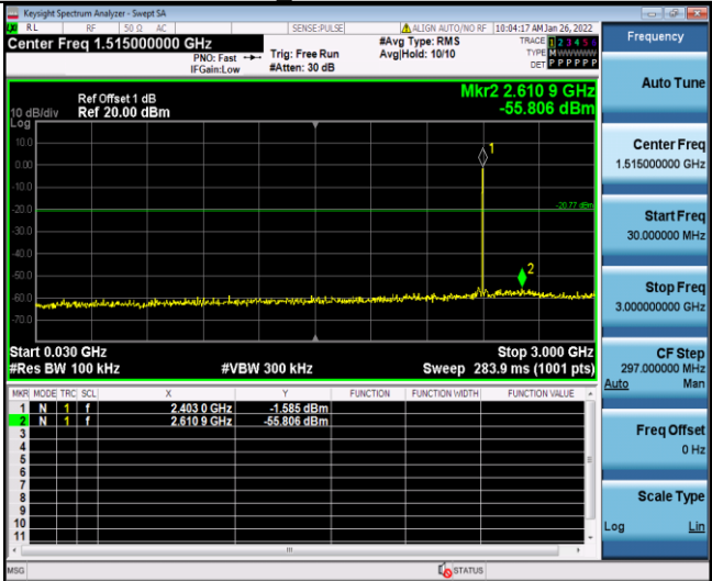
BLE 2402 30-3000
