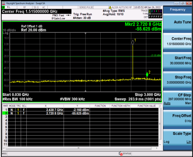
BLE 2440 30-3000
