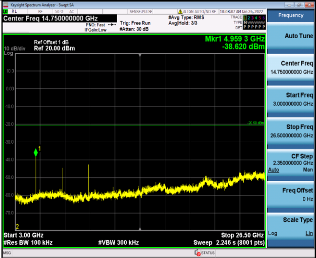
BLE 2480 3000-26500
