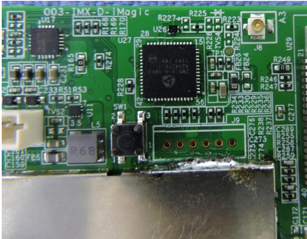
Z-wave module
