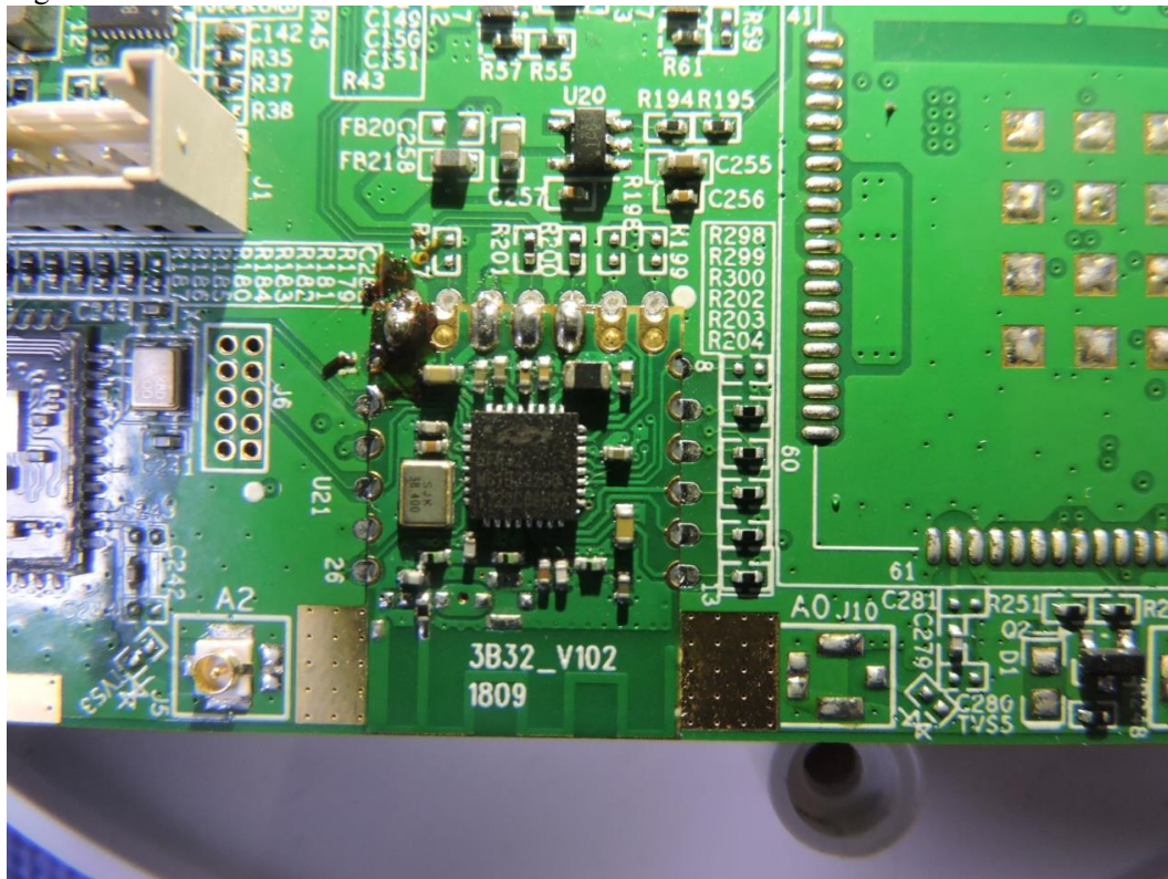
Zigbee module
