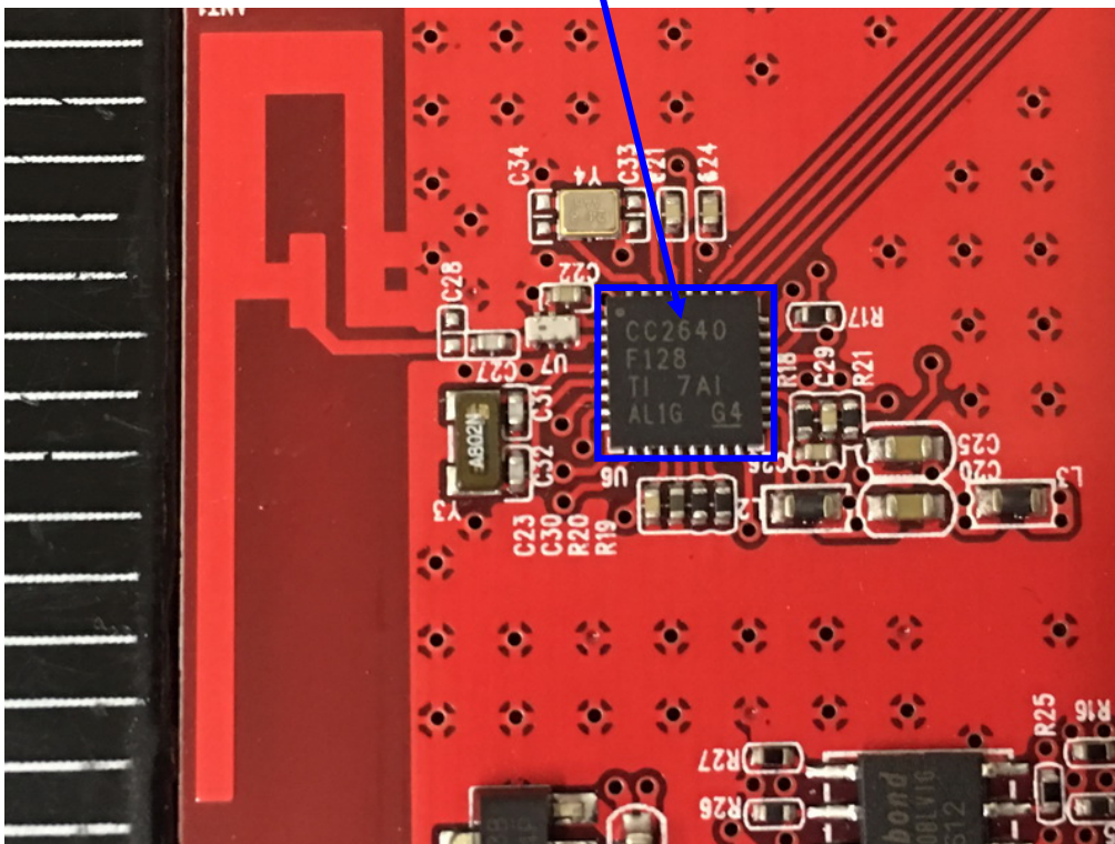
BLE RF Chip IC – Top View
