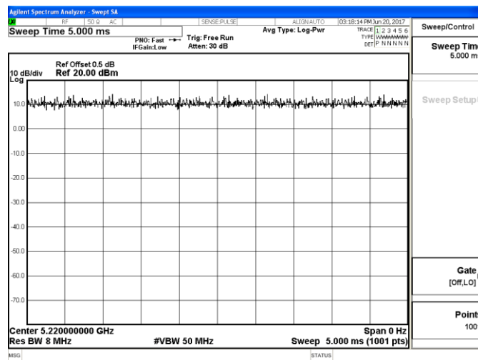
n20-5220MHz
