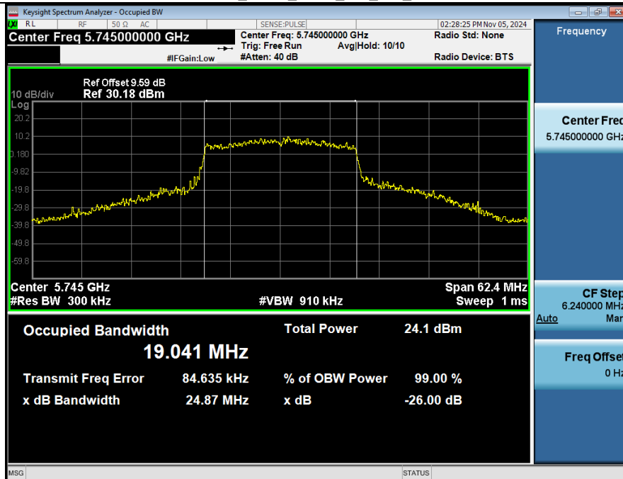
99% OCB NVNT ANT2 802 11a 5745
