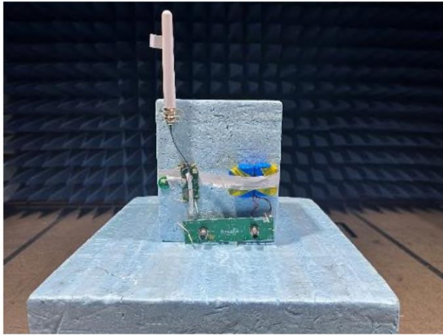
EUT Upright
