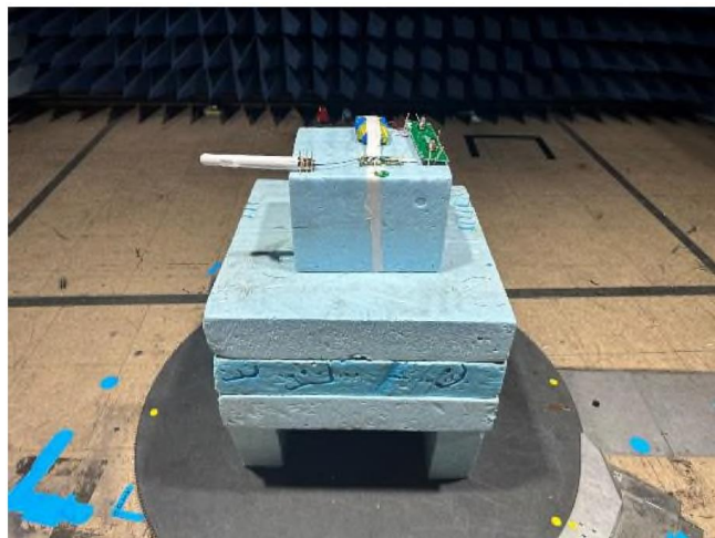
EUT Flat
