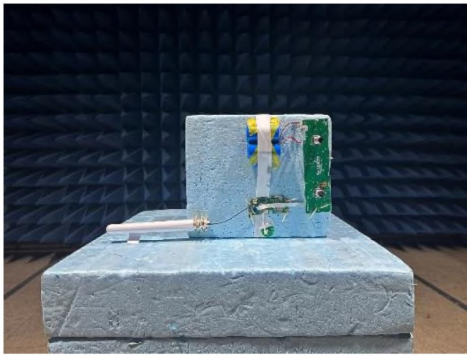
EUT Side
