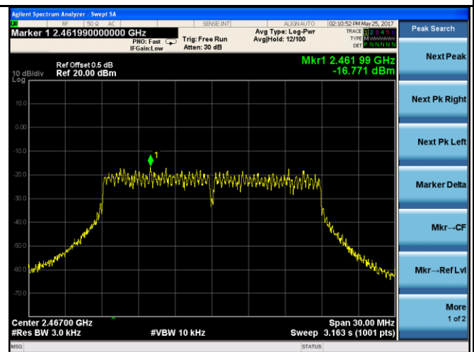
PSD - CH 12 - 802.11n20
