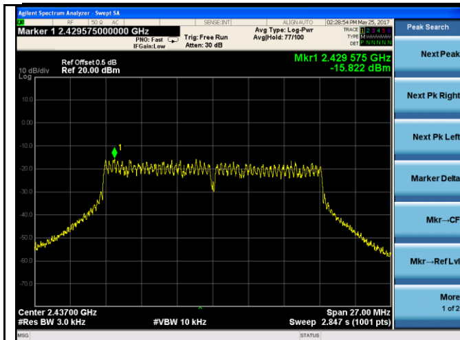
PSD - CH 6 - 802.11g
