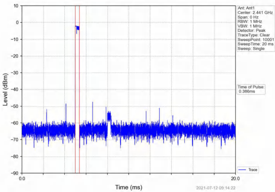
\pi /4-DQPSK_2DH1_HOPP_Ant1_NTNV
