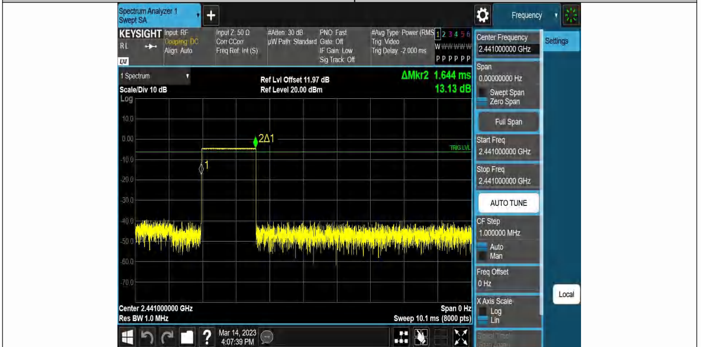
DH3-Ant1-Hop-1.644-160
