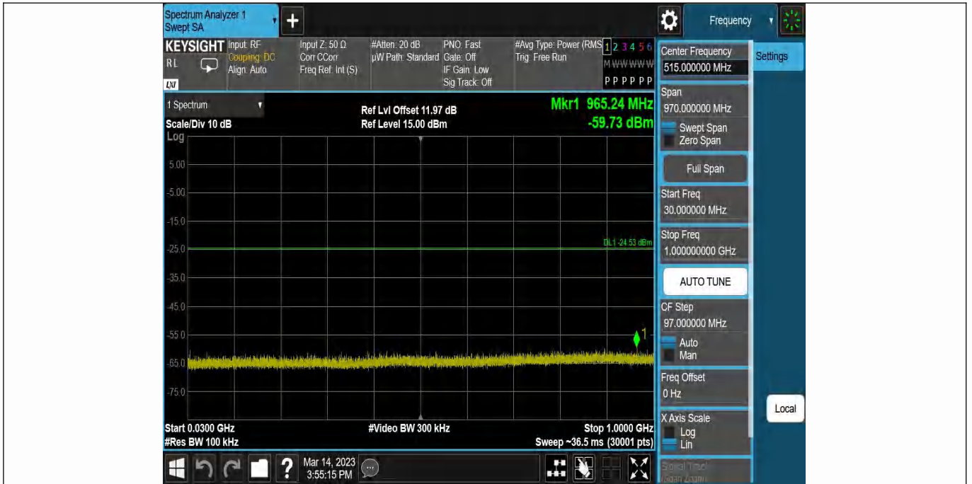
DH5-Ant1-2441-30~1000--4.53
