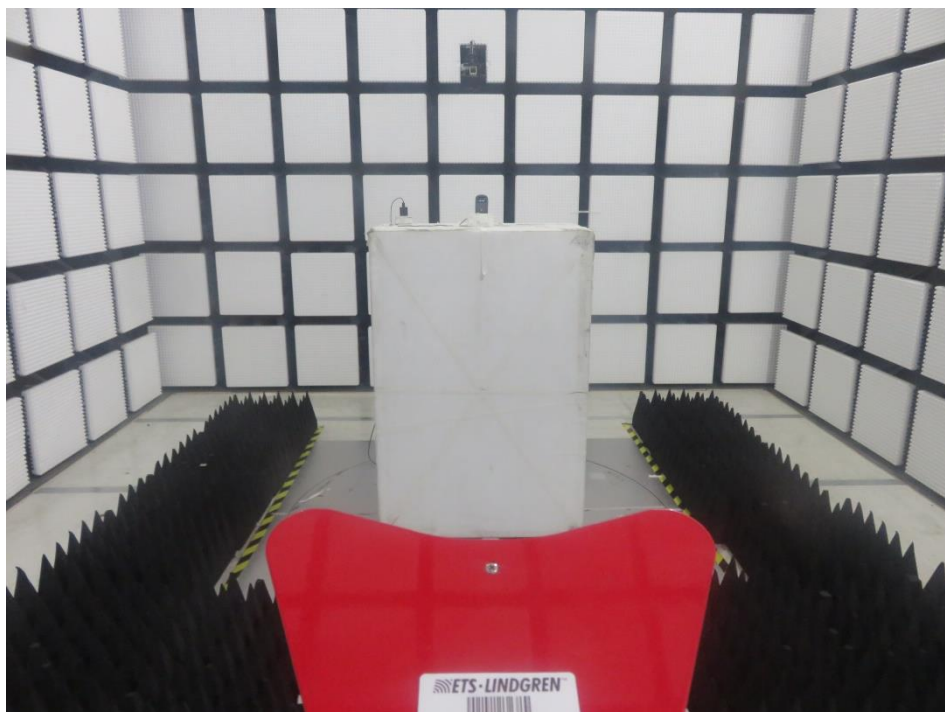
1610~10600MHz @3m
