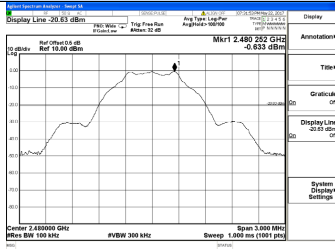
2479 – 2481 MHz
