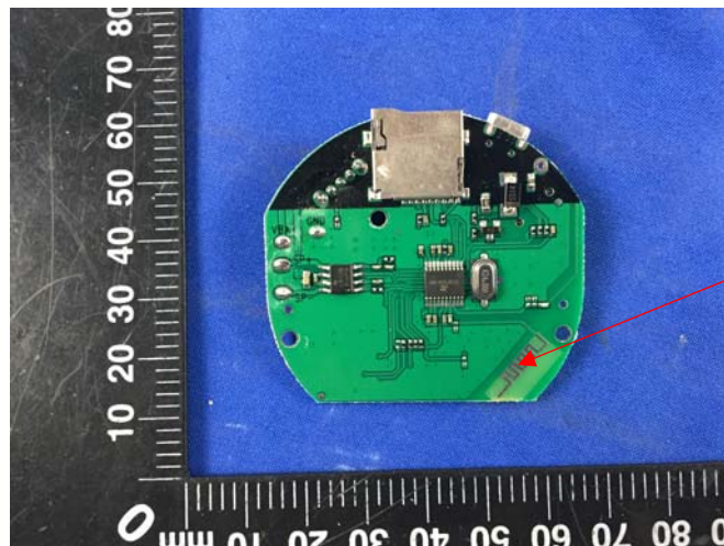
Antenna
