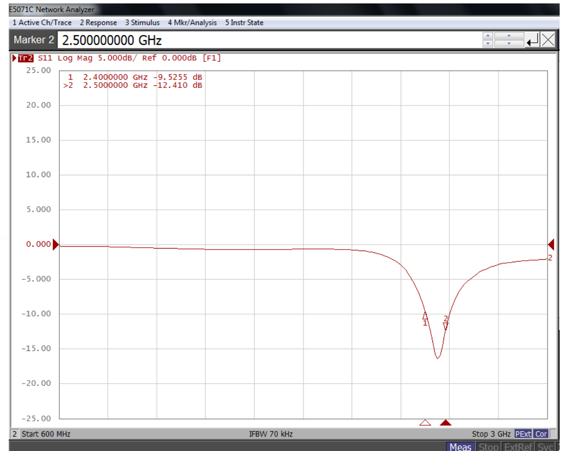
S-Parameter Test
