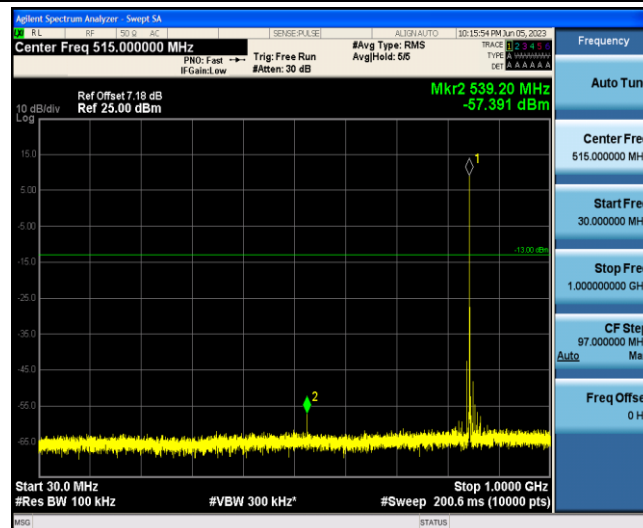
Band5-3MHz-QPSK-20635-1-0-Low-30-1000--57.39-PASS
