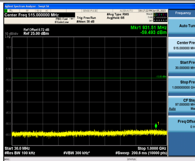
Band2-20MHz-QPSK-18900-1-0-Low-30-1000--59.49-PASS
