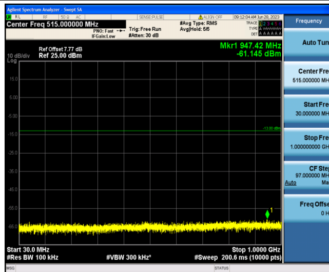
Band4-3MHz-QPSK-19965-1-0-Low-30-1000--61.15-PASS
