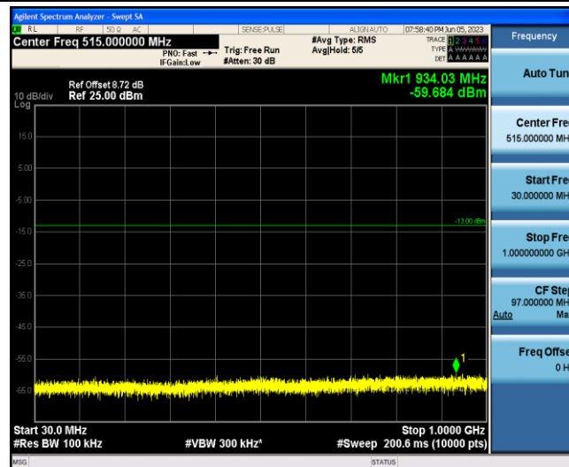
Band2-5MHz-QPSK-18900-1-0-Low-30-1000--59.68-PASS
