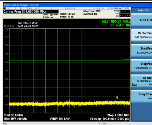
Band2-1.4MHz-QPSK-18900-1-0-Low-30-1000--59.2-PASS
