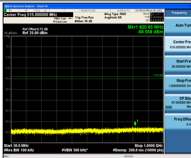
Band2-5MHz-16QAM-18900-1-0-Low-30-1000--59.56-PASS
