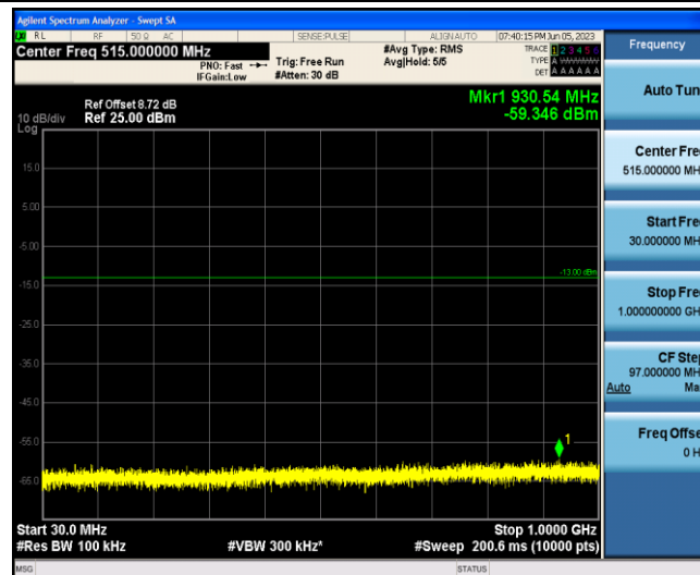
Band2-3MHz-16QAM-18900-1-0-Low-30-1000--59.35-PASS
