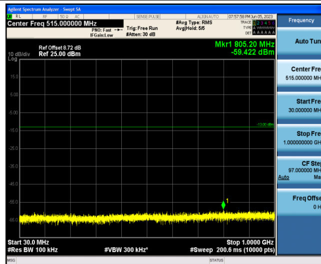
Band2-5MHz-QPSK-18625-1-0-Low-30-1000--59.42-PASS
