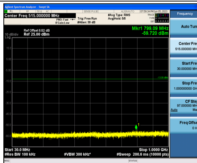
Band2-5MHz-QPSK-19175-1-0-Low-30-1000--59.72-PASS
