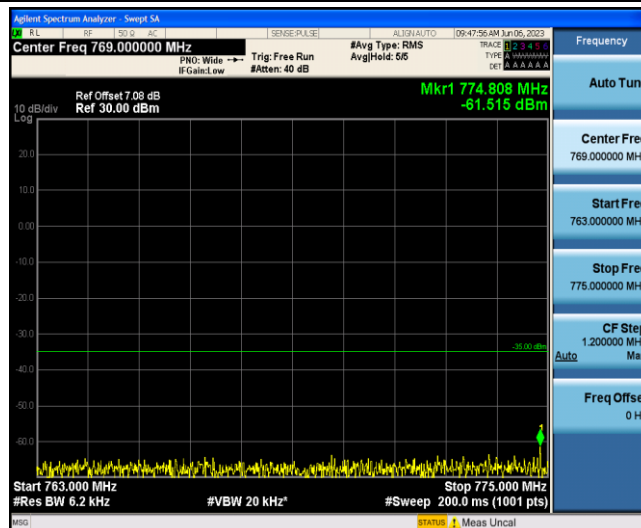
Band13-10MHz-QPSK-23230-1-0-Low-763-775--61.52-PASS
