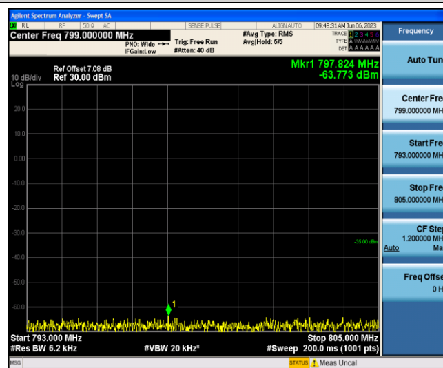
Band13-10MHz-16QAM-23230-1-0-Low-793-805--63.77-PASS
