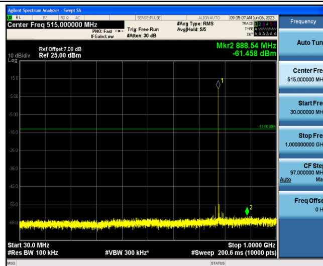
Band13-5MHz-QPSK-23230-1-0-Low-30-1000--61.46-PASS
