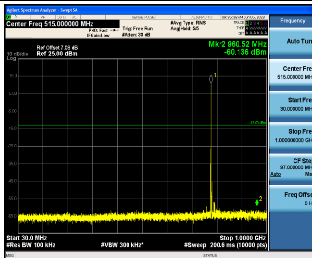
Band13-5MHz-16QAM-23255-1-0-Low-30-1000--60.14-PASS
