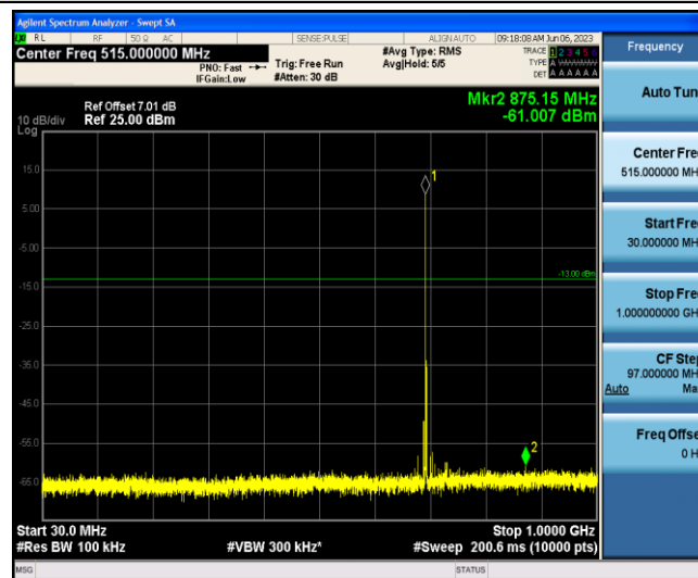
Band12-10MHz-16QAM-23060-1-0-Low-30-1000--61.01-PASS
