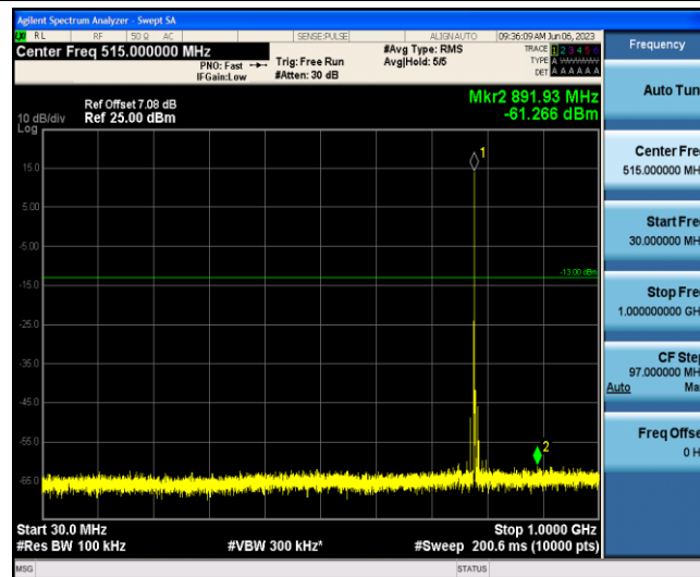
Band13-5MHz-QPSK-23255-1-0-Low-30-1000--61.27-PASS
