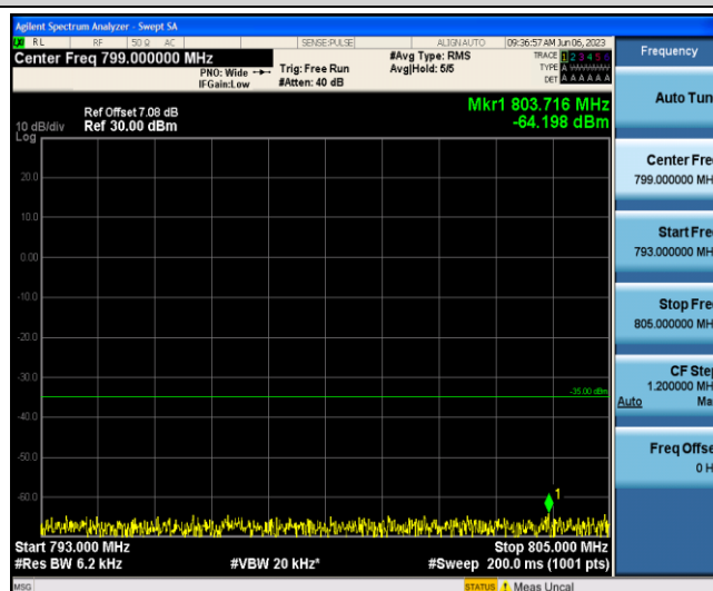
Band13-5MHz-16QAM-23255-1-0-Low-793-805--64.2-PASS
