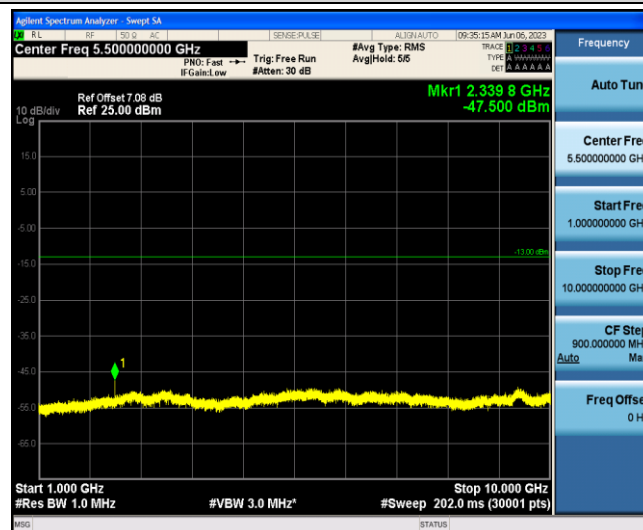
Band13-5MHz-QPSK-23230-1-0-Low-1000-10000--47.5-PASS
