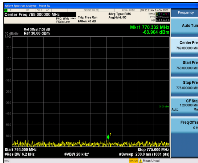
Band13-5MHz-QPSK-23230-1-0-Low-763-775--63.9-PASS
