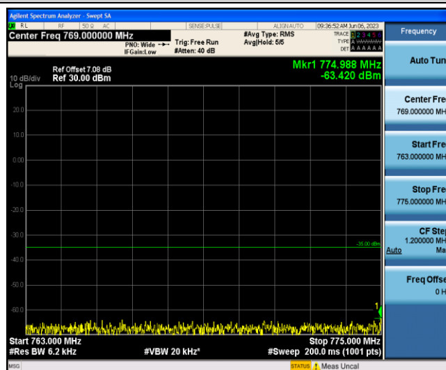
Band13-5MHz-16QAM-23255-1-0-Low-763-775--63.42-PASS
