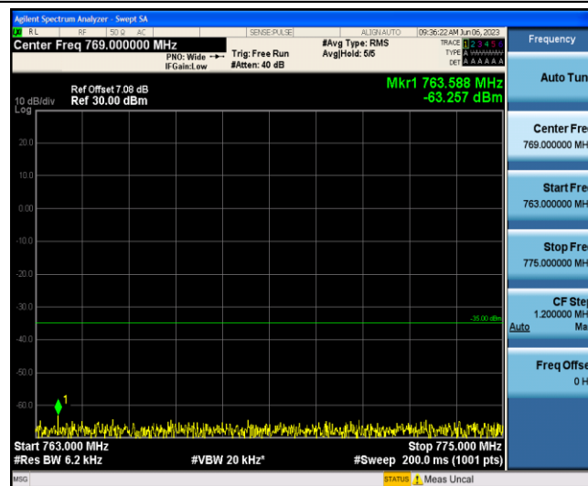
Band13-5MHz-QPSK-23255-1-0-Low-763-775--63.26-PASS
