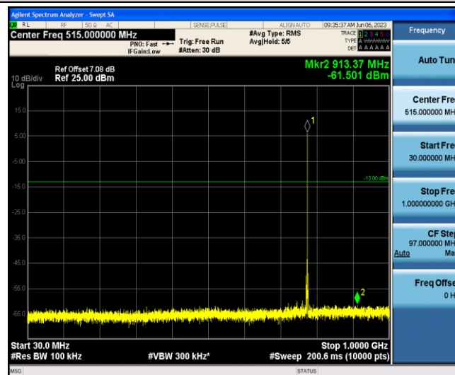
Band13-5MHz-16QAM-23230-1-0-Low-30-1000--61.5-PASS
