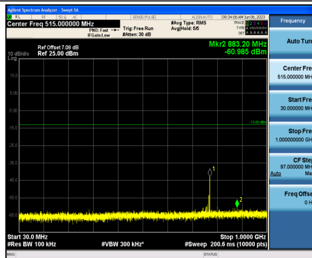
Band13-5MHz-QPSK-23205-1-0-Low-30-1000--60.99-PASS
