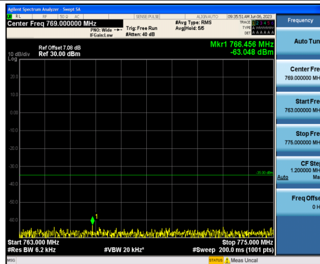
Band13-5MHz-16QAM-23230-1-0-Low-763-775--63.05-PASS
