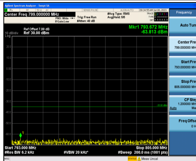
Band13-5MHz-16QAM-23205-1-0-Low-793-805--63.81-PASS
