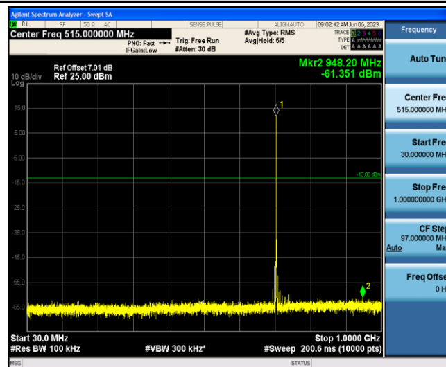
Band12-5MHz-QPSK-23155-1-0-Low-30-1000--61.35-PASS
