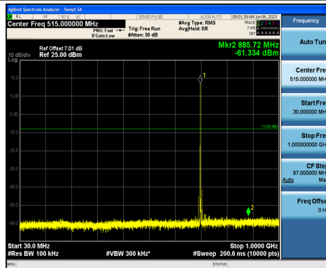
Band12-5MHz-QPSK-23095-1-0-Low-30-1000--61.33-PASS
