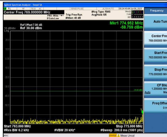
Band13-5MHz-16QAM-23205-1-0-Low-763-775--59.76-PASS
