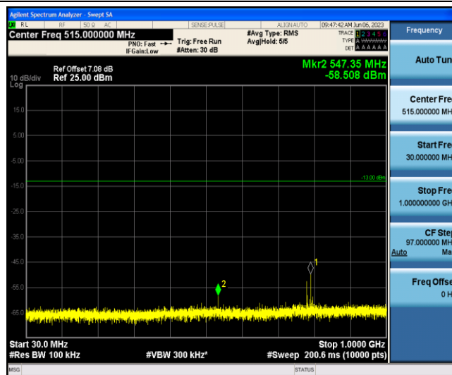
Band13-10MHz-QPSK-23230-1-0-Low-30-1000--58.51-PASS
