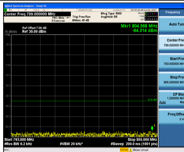
Band13-5MHz-QPSK-23230-1-0-Low-793-805--64.01-PASS
