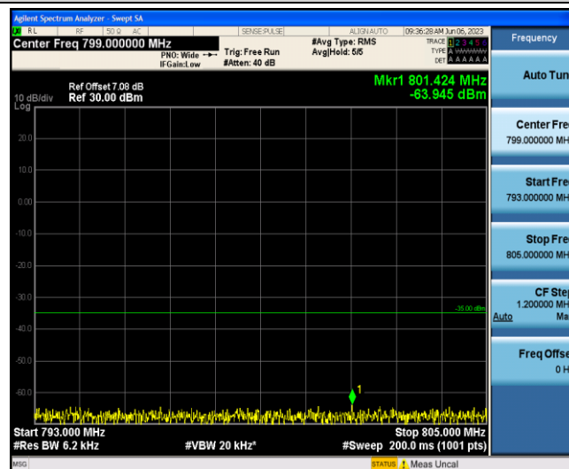
Band13-5MHz-QPSK-23255-1-0-Low-793-805--63.95-PASS
