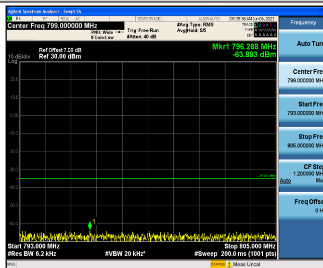
Band13-5MHz-16QAM-23230-1-0-Low-793-805--63.89-PASS
