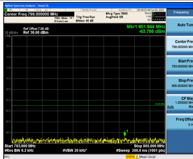
Band13-10MHz-QPSK-23230-1-0-Low-793-805--63.77-PASS
