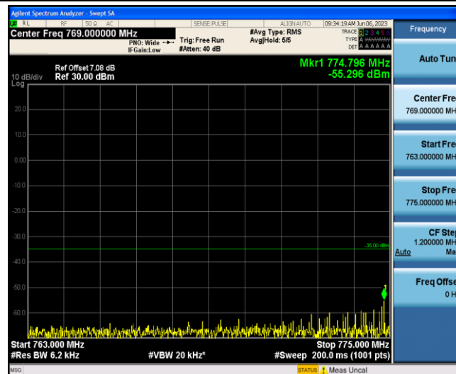
Band13-5MHz-QPSK-23205-1-0-Low-763-775--55.3-PASS
