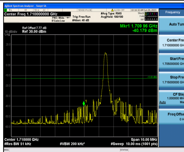
Band4-20MHz-QPSK-20050-1-0-Low--40.18-PASS
