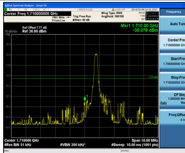
Band4-10MHz-QPSK-20000-1-0-Low--35.08-PASS
