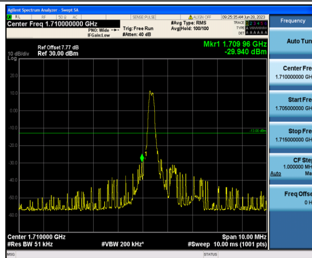
Band4-5MHz-QPSK-19975-1-0-Low--29.94-PASS
