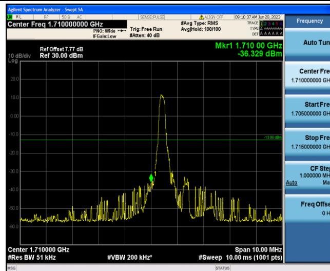
Band4-3MHz-QPSK-19965-1-0-Low--36.33-PASS
