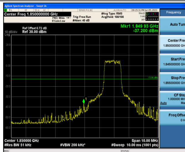
Band2-20MHz-QPSK-18700-6-0-Low--37.20-PASS
