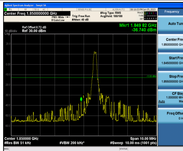
Band2-10MHz-QPSK-18650-1-0-Low--36.74-PASS
