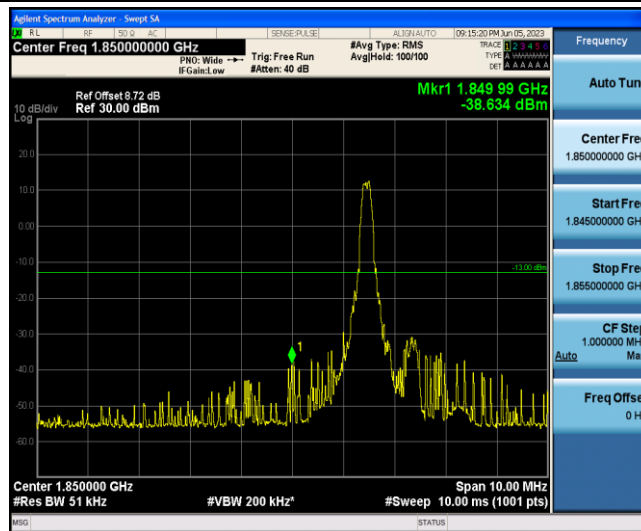
Band2-20MHz-16QAM-18700-1-0-Low--38.63-PASS
