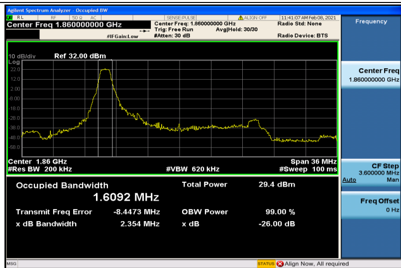
Band2-20MHz-16QAM-18700-6RB#0-1.6092
