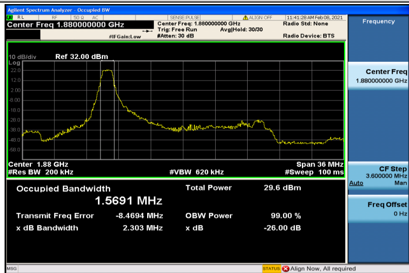
Band2-20MHz-16QAM-18900-6RB#0-1.5691
