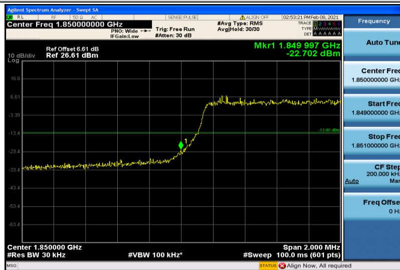
Band2-3MHz-QPSK-18615-6RB#0
