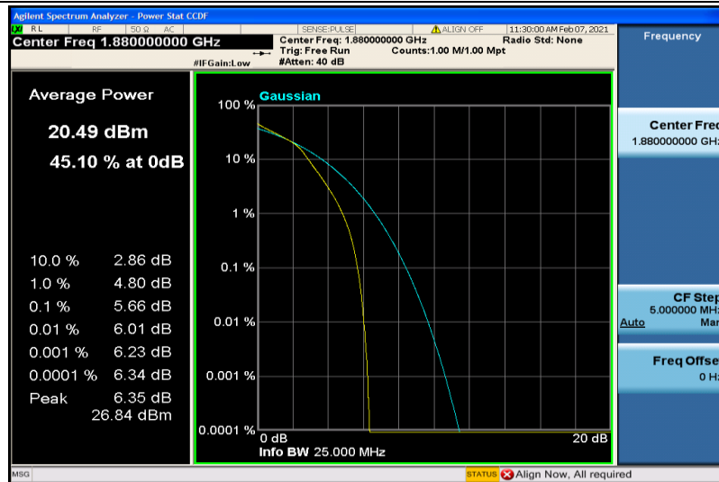
Band2-3MHz-16QAM-18900-6RB#0
