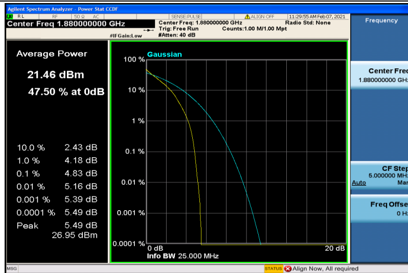
Band2-3MHz-QPSK-18900-6RB#0
