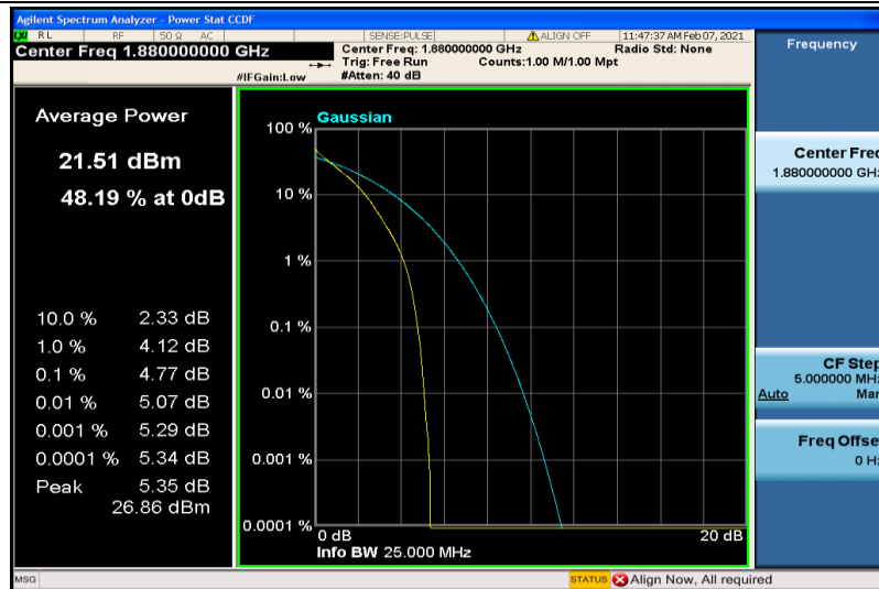
Band2-5MHz-QPSK-18900-6RB#0
