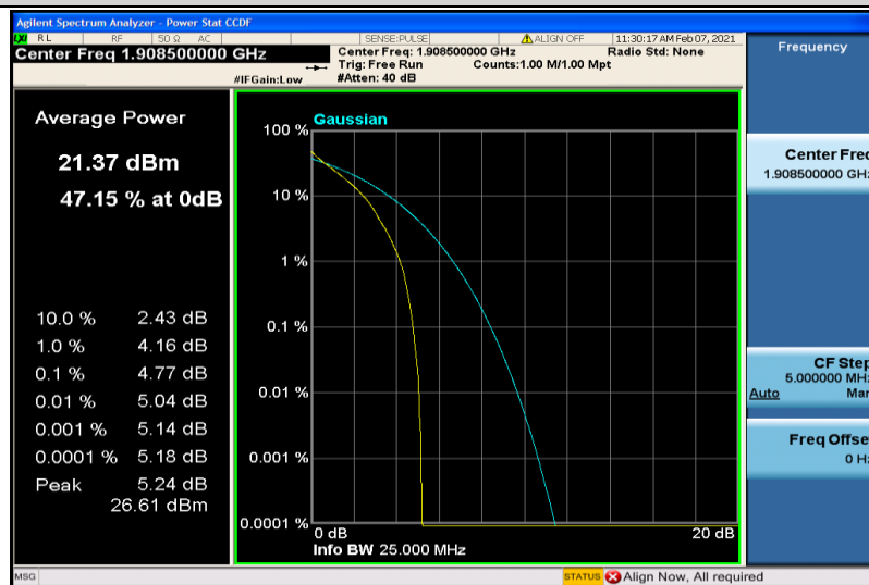
Band2-3MHz-QPSK-19185-6RB#0
