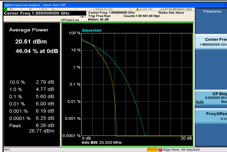
Band2-5MHz-16QAM-18900-6RB#0
