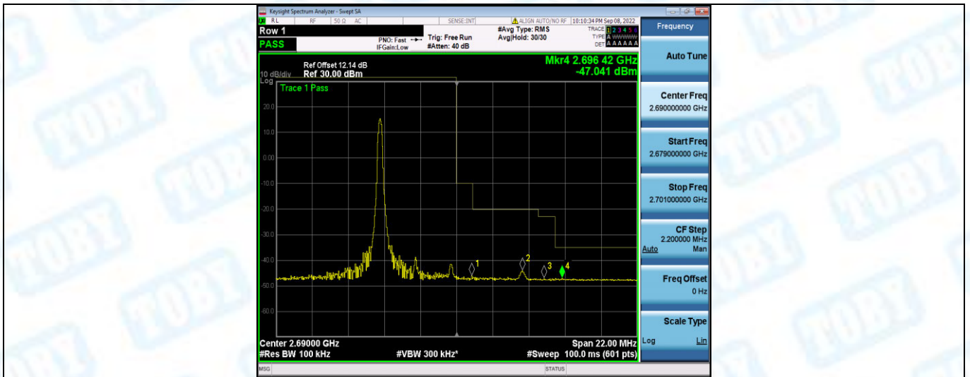
Band41-5MHz-16QAM-41565-1RB#24
